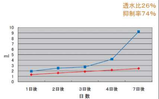
図-4 促進膨張試験結果
