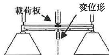
試験状況図
