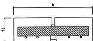
試験体概略図 (製品名: マチスリット側溝 300 F 型)
