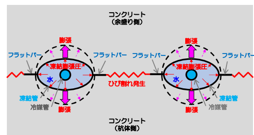
図-2 凍結膨張圧によるひび割れ発生のおき
