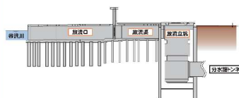
段面図
