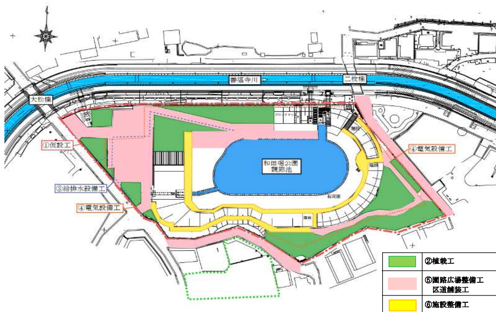
全体平面図
