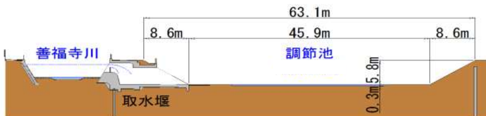
断面図
