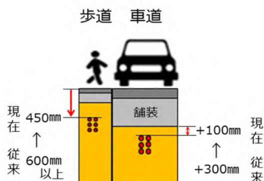
図 11-2 浅層埋設のイメージ
