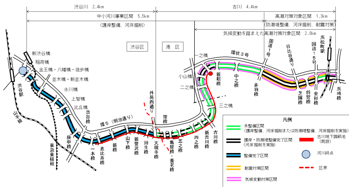
図4-1 渋谷川・古川河川整備箇所図
