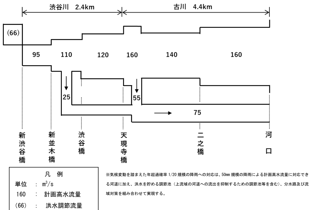
図 3－1 渋谷川・古川計画流量配分図
