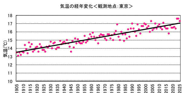
図 1-4 東京の年平均気温経年変化 (1905~2025 年)
