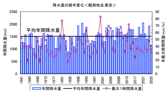
図 1-3 東京の年間降水量、最大時間雨量経年変化 (1961~2025 年)
