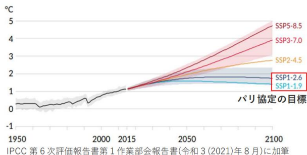
図 1-6 1850年~1900年を基準とした世界平均気温の変化
