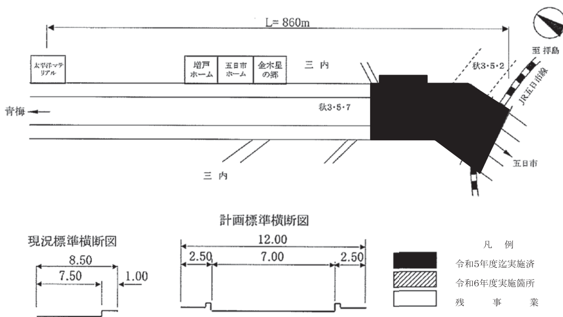
主31号(三内地区)整備状況図
