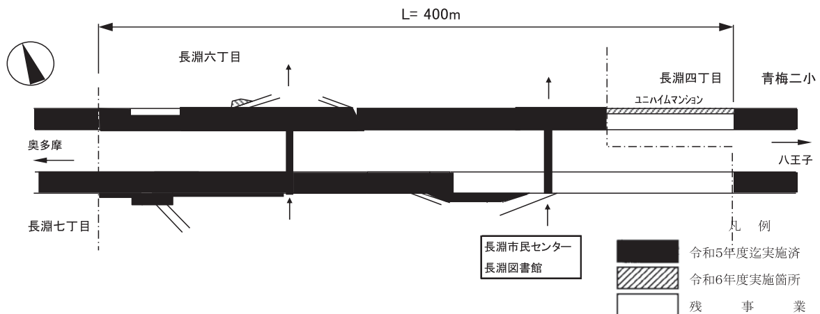
国道411号(長淵4～6丁目地区)整備状況図
