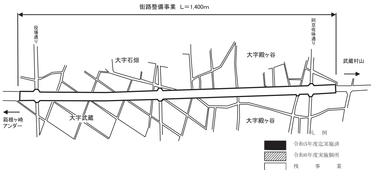
福生3・4・4号 整備状況図
