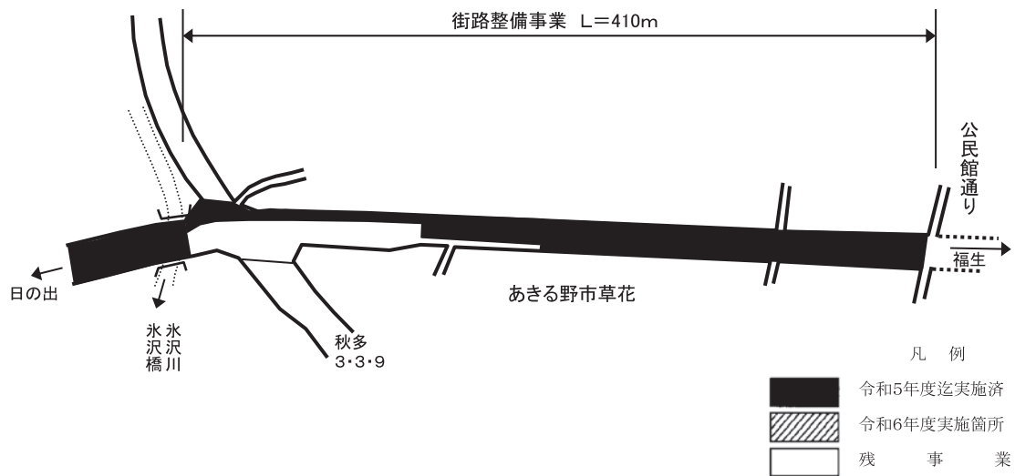
秋多3・4・6号(第四工区) 整備状況図
