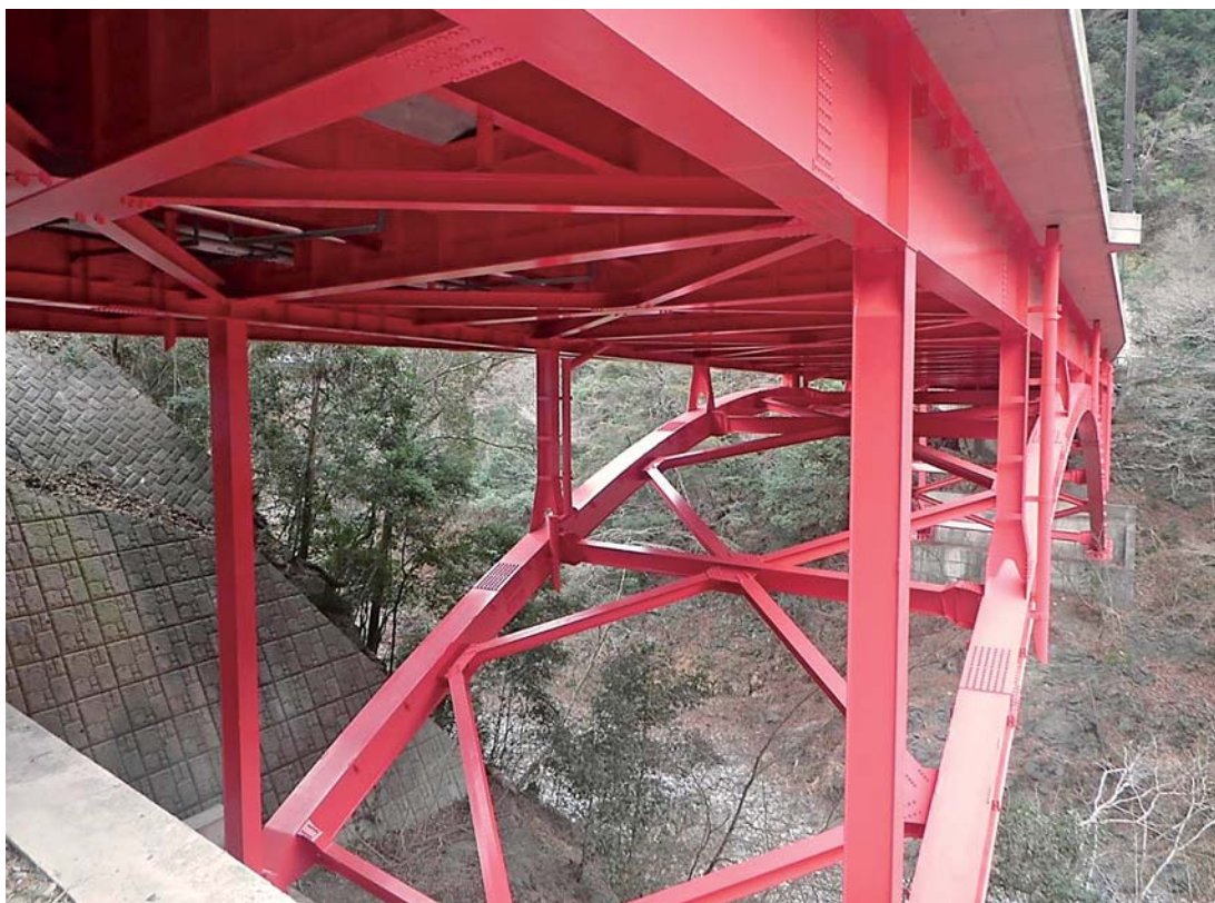
橋梁維持事業（愛宕大橋塗装） 「一般都道奥多摩あきる野線（第184号）多摩川南岸道路」 西多摩郡奥多摩町氷川地内 平成31年2月完成
