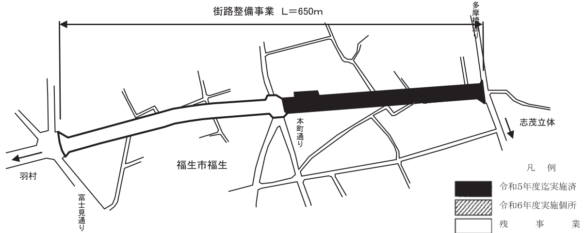
福生3・3・30号 整備状況図
