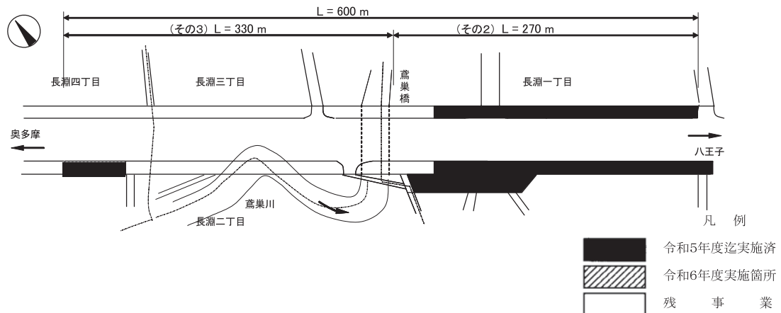
国道411号(長淵1～3丁目地区)整備状況図
