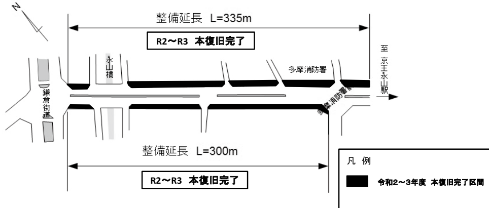
図-26 電線共同溝整備 主18府中町田線（永山駅周辺）
