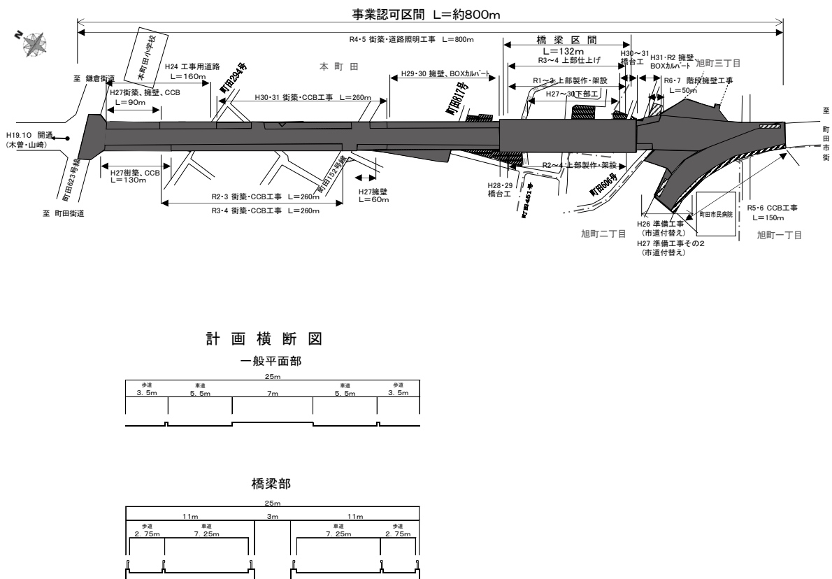
図-18 町田3・3・36号〔旭町〕（相原鶴間線）
