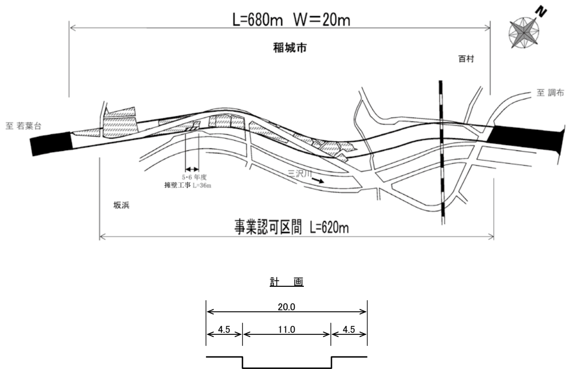
図-17 町田調布線（主19号 鶴川街道）百村
