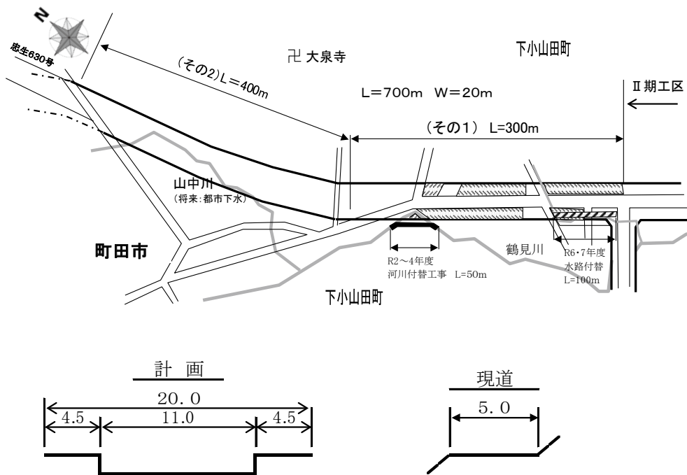
図-15 町田平山八王子線（一155号）図師・下小山田地区：図師Ⅲ期
