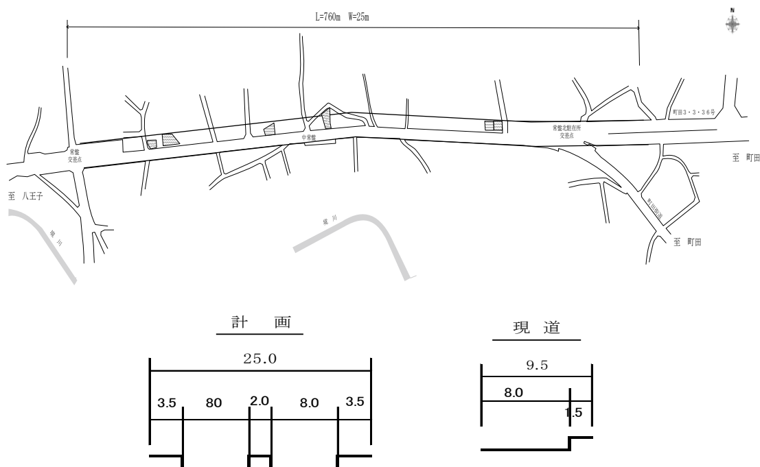
図-12 主要地方道八王子町田線（主47号 町田街道）常盤町地区
