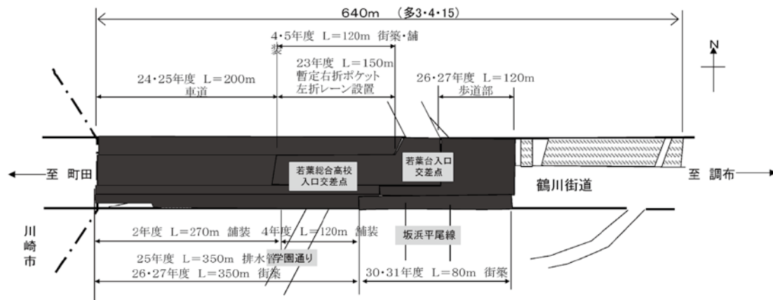
図-22 自歩道坂浜（電共若葉総合高校入口）
