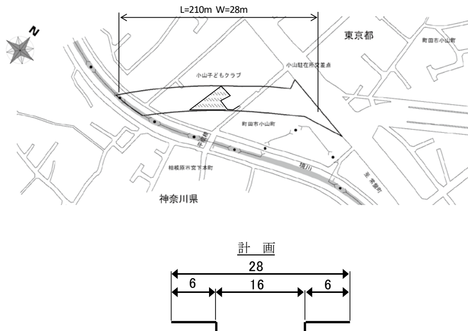
図-16 相模原立川線（一503号）小山町地区：南多摩尾根幹線延伸部
