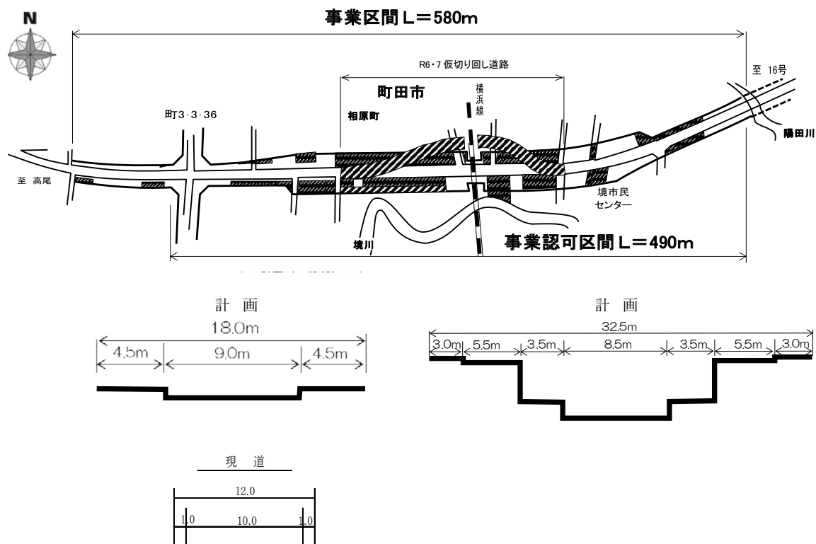
図-13 主要地方道八王子町田線（主47号 町田街道）相原地区
