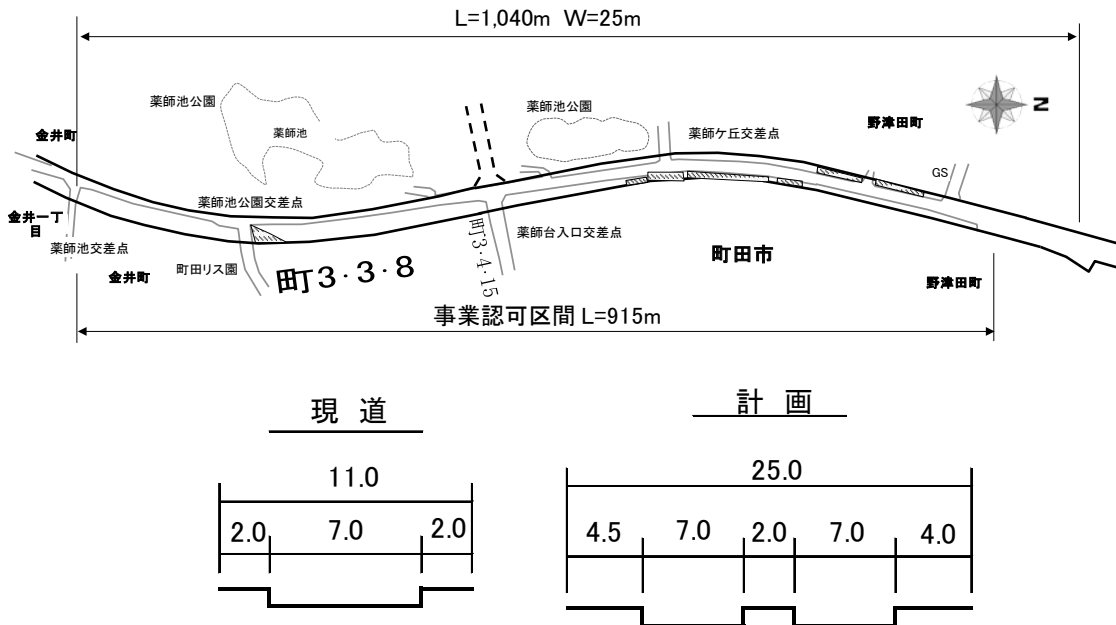
図-11 主要地方道府中町田線（主18号 鎌倉街道）薬師池Ⅱ期
