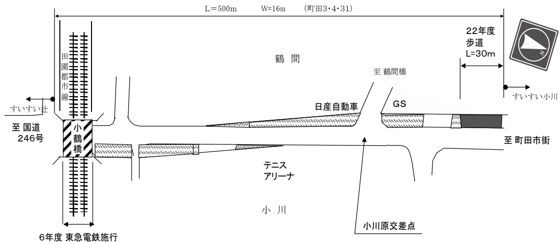
図-24 第3次交差点すいすいプラン [小川原]
