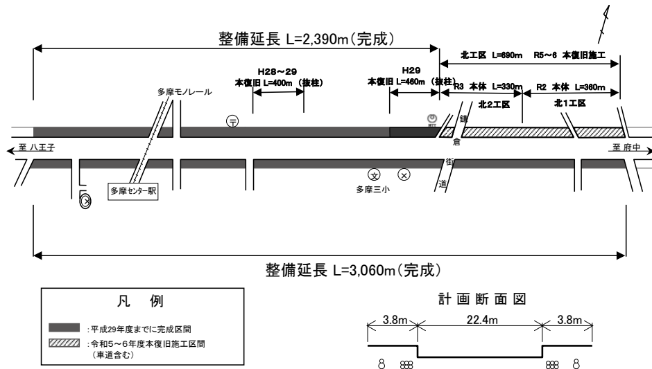
図-25 電線共同溝整備 都158小山乞田線（多摩ニュータウン通り）及び主18府中町田線（鎌倉街道：北工区）
