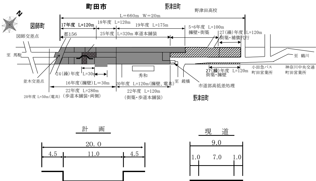
図-14 主要地方道相模原大蔵町線（主57号 芝溝街道）並木地区
