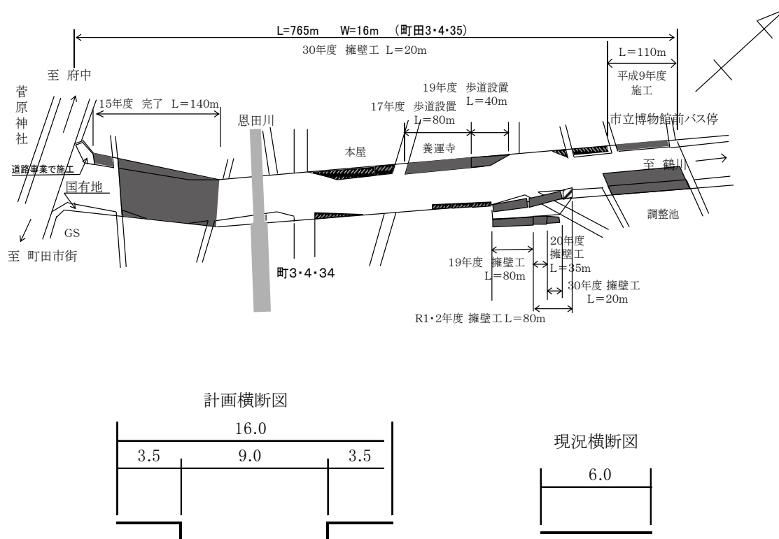
図-21 世田谷町田線（主3号 鶴川街道）玉川学園
