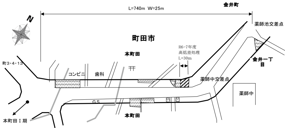
図-10 主要地方道府中町田線（主18号 鎌倉街道）薬師池Ⅰ期
