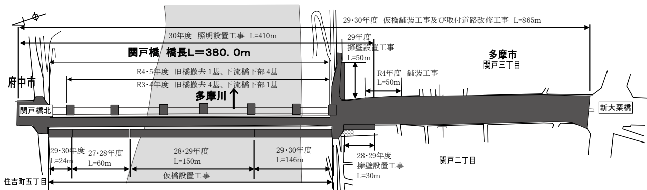
図-20 府中町田線（主18号 鎌倉街道）関戸橋
