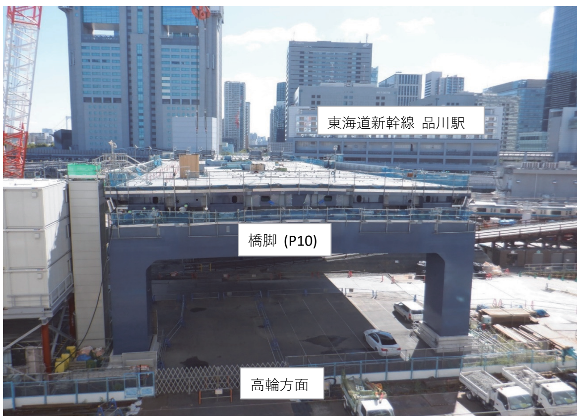
〔街路整備〕環状第4号線 鉄道区域施工状況(鉄道会社協定委託工事)上部工施行中
