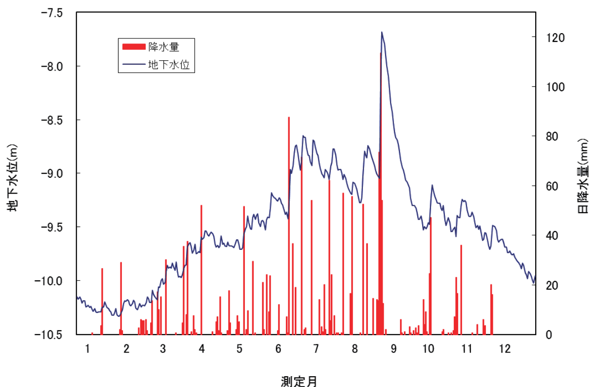
図-3 2024 年地下水位と降水量 ①中野区 新井 北野神社
