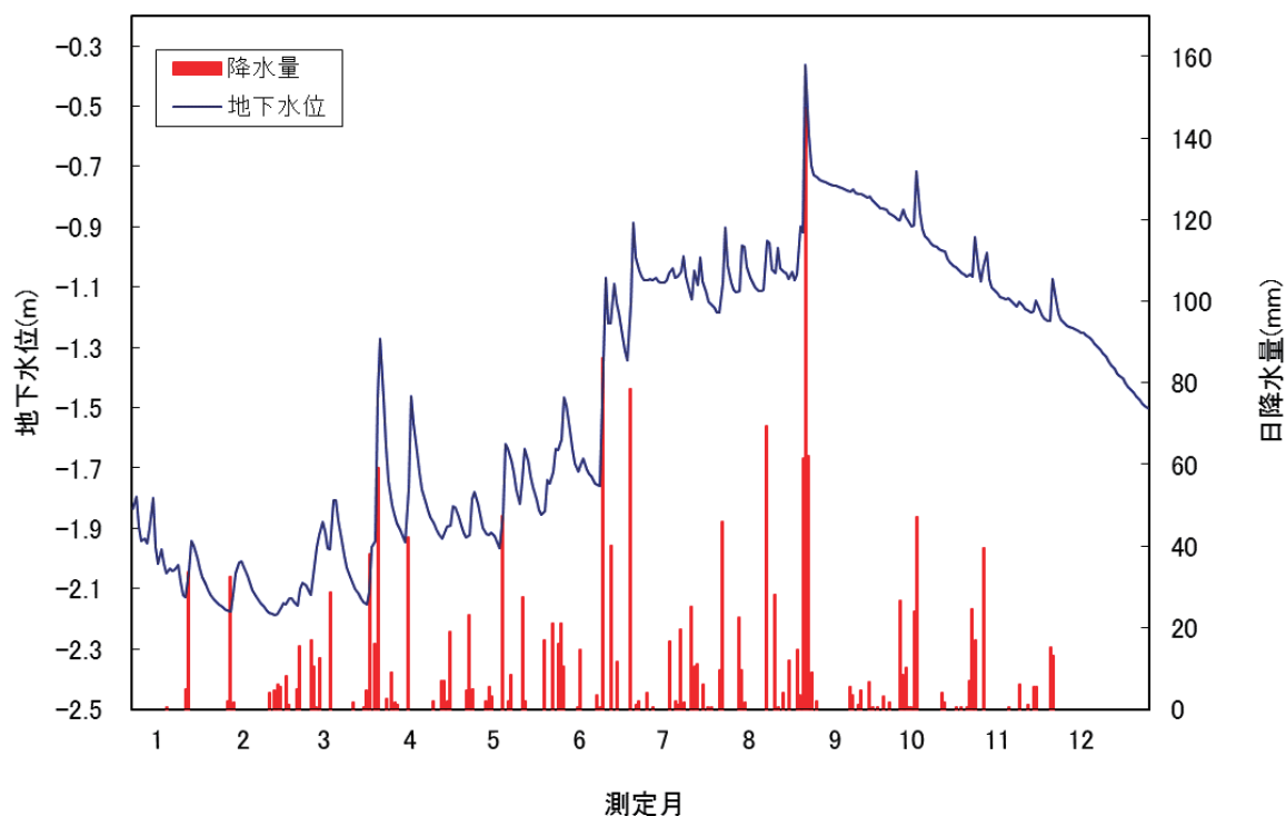
図－6 2024 年地下水位と降水量 ④′府中市 多磨町
