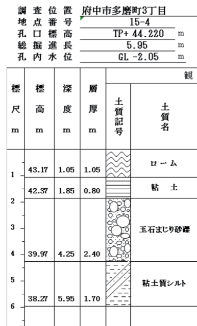
図—9 観測井柱状図（府中市・多磨町）
