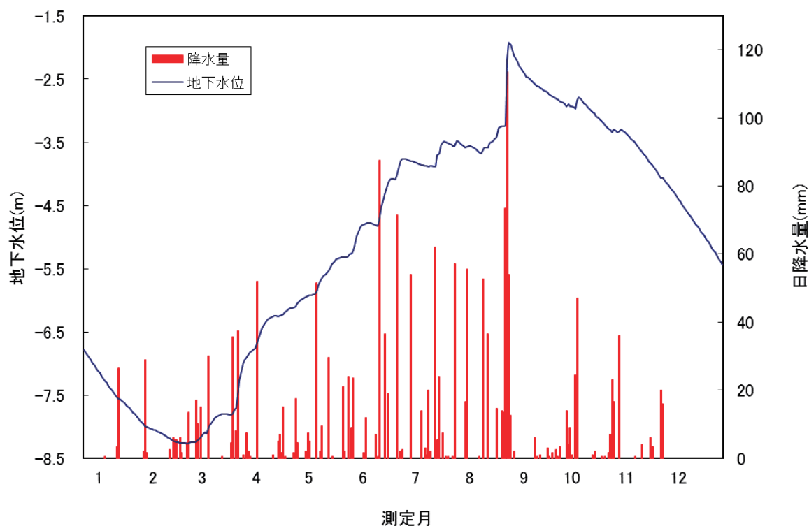
図－4 2024 年地下水位と降水量 ②東久留米市 小平霊園
