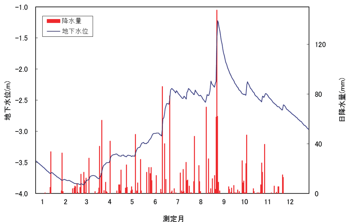
図－5 2024 年地下水位と降水量 ③三鷹市 井の頭公園
