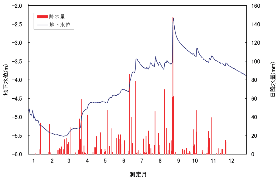
図ー7 2024 年地下水位と降水量 ⑤小金井市 前原
