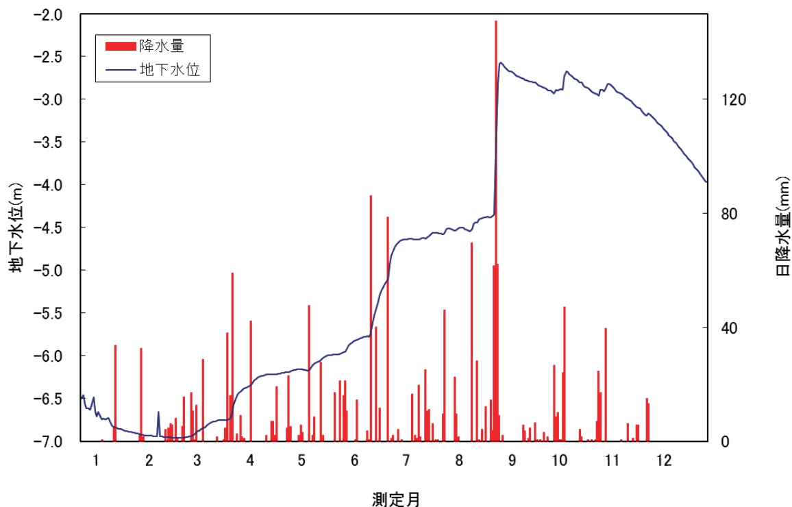
図一8 2024 年地下水位と降水量 ⑥小金井市 貫井南町
