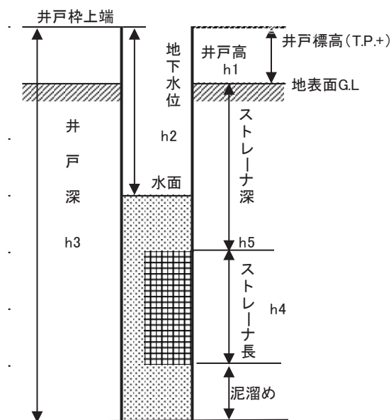
図-2 地下水位測定要素
