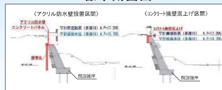
標準断面図
