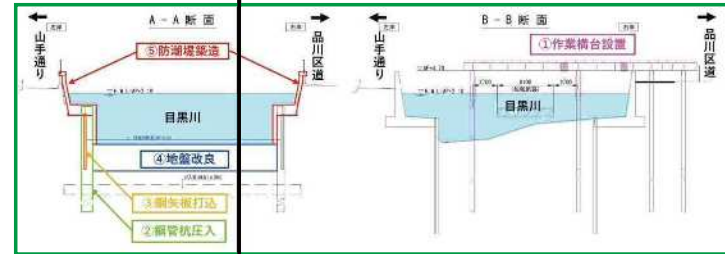
断面図
