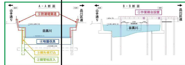
断面図
