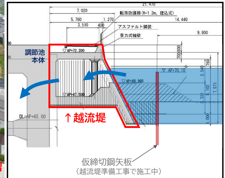
横断図
