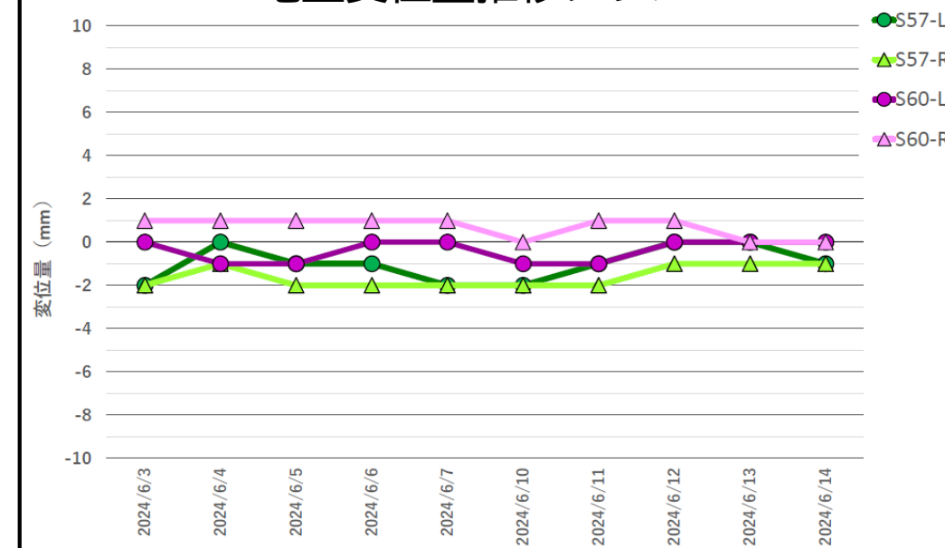
地盤変位量推移グラフ
