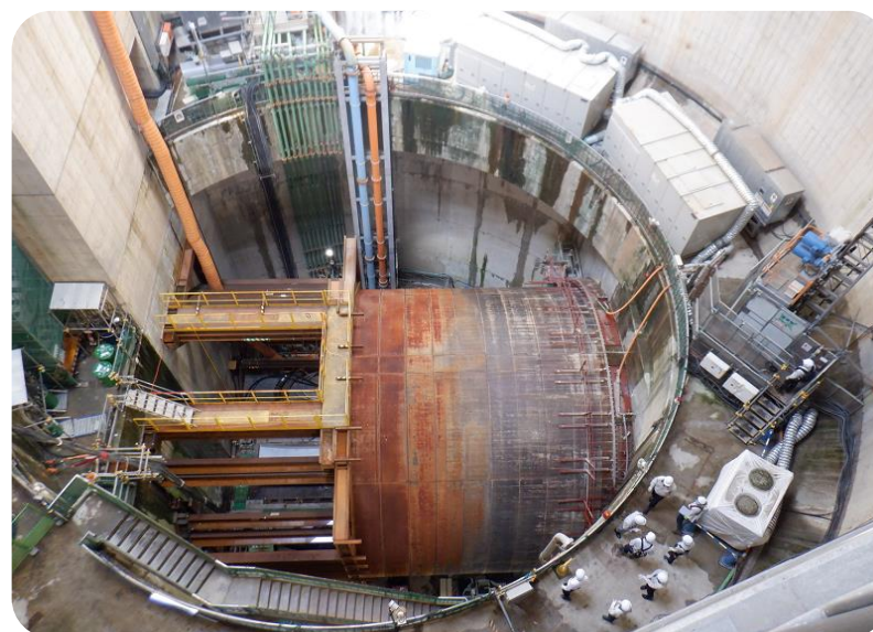
発進立坑からシールドマシン発進状況
