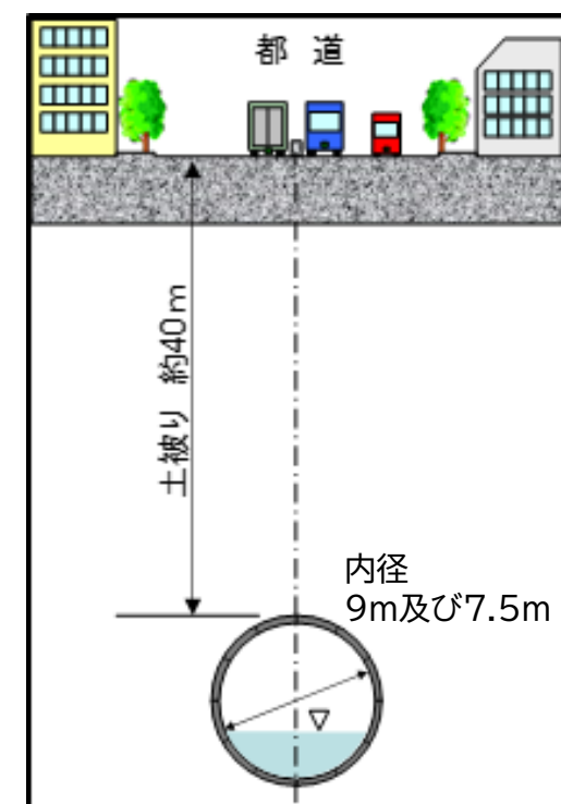
断面図
