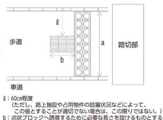
図 4-10 踏切道手前の設置例
