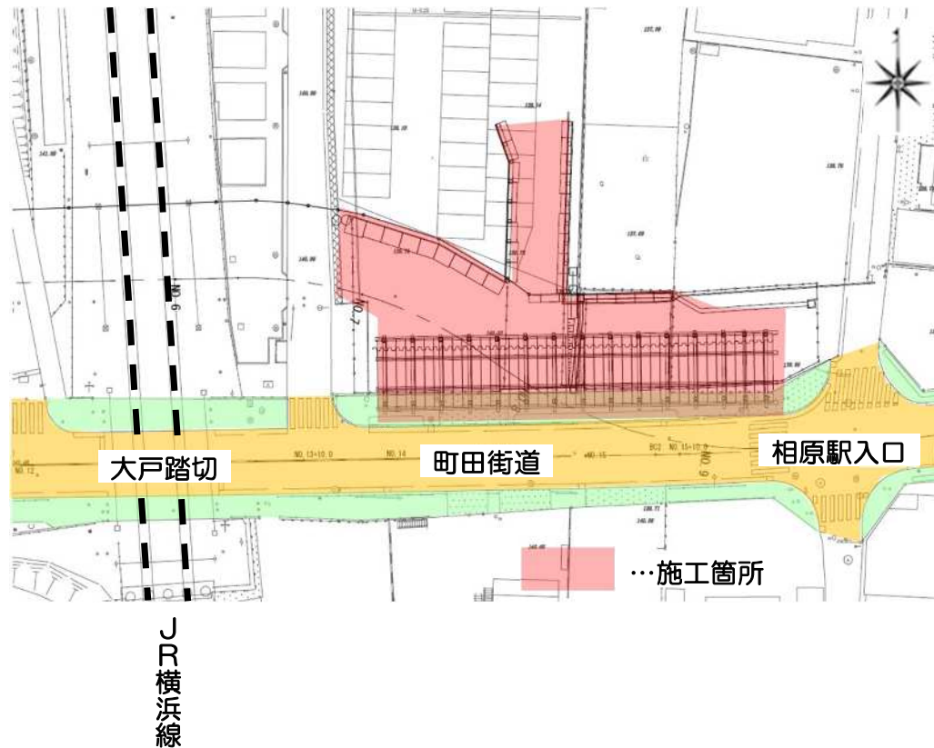
《計画平面図》
