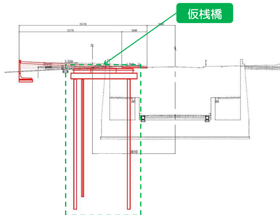
《計画断面図》
