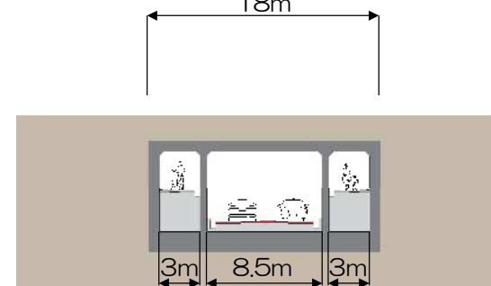
B-B断面（鉄道横断部）
