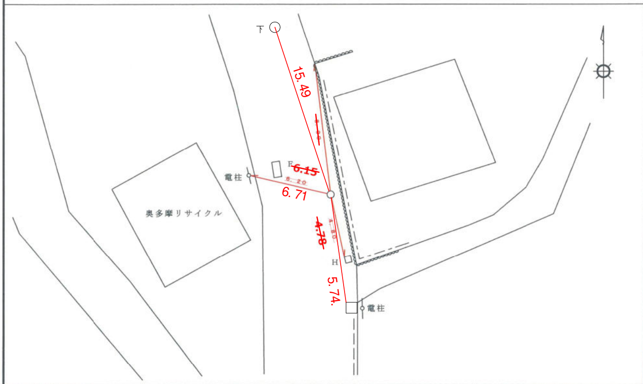
詳 細 図
