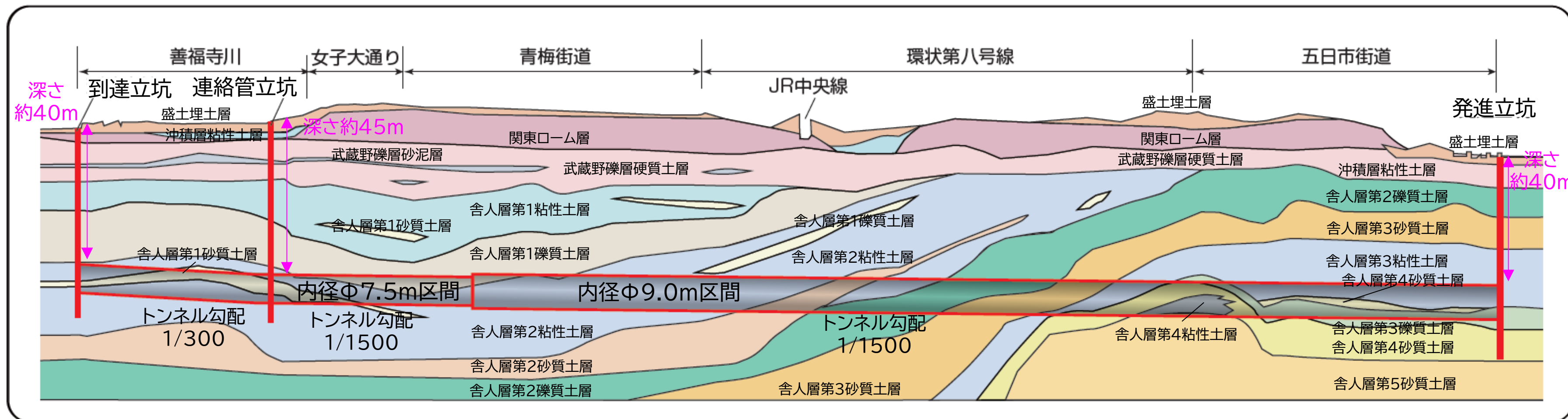
【地質調査から推定した地質縦断図とトンネル設置箇所】
