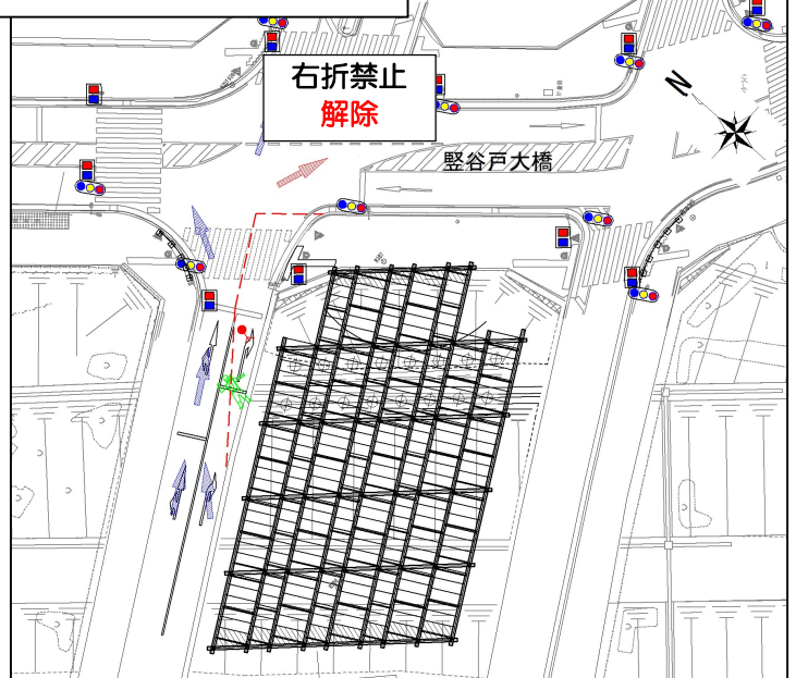
豎谷戸大橋交差点拡大図
