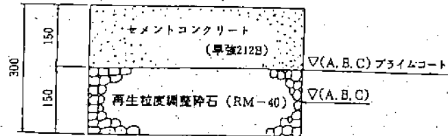
歩道乗入れ舗装（セメコン） 30型
