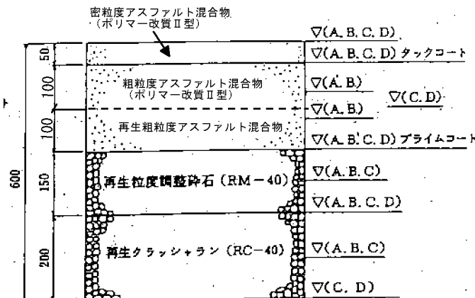
アスファルトコンクリート舗装 60型
