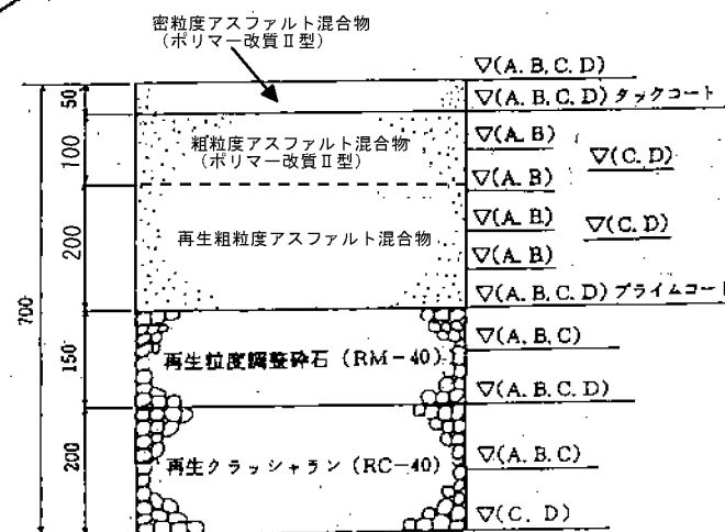
アスファルトコンクリート舗装 70型
