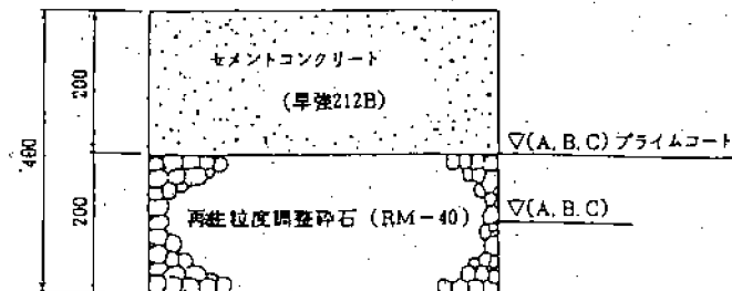
歩道乗入れ舗装（セメコン） 40型
