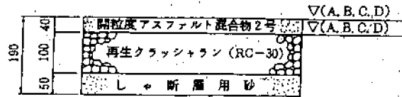
アスファルトコンクリート舗装（透水性）
