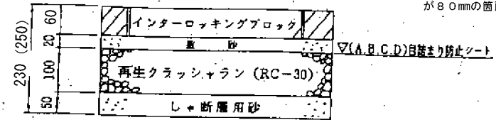
歩道インターロッキングブロック舗装（透水性）
