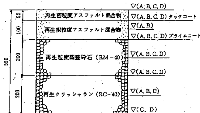
アスファルトコンクリート舗装 55型
