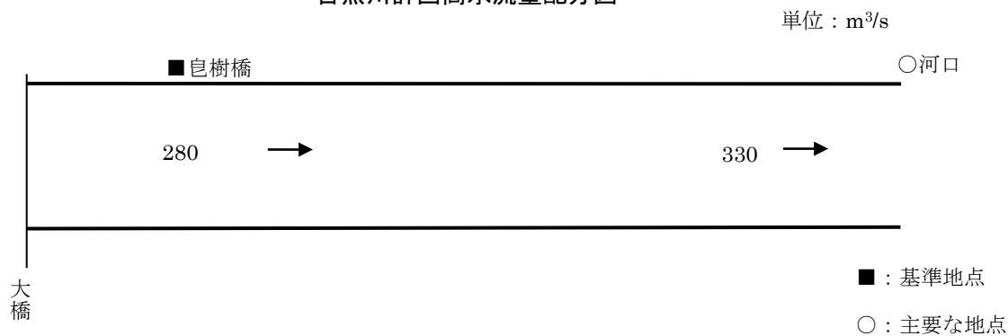
目黒川計画高水流量配分図
