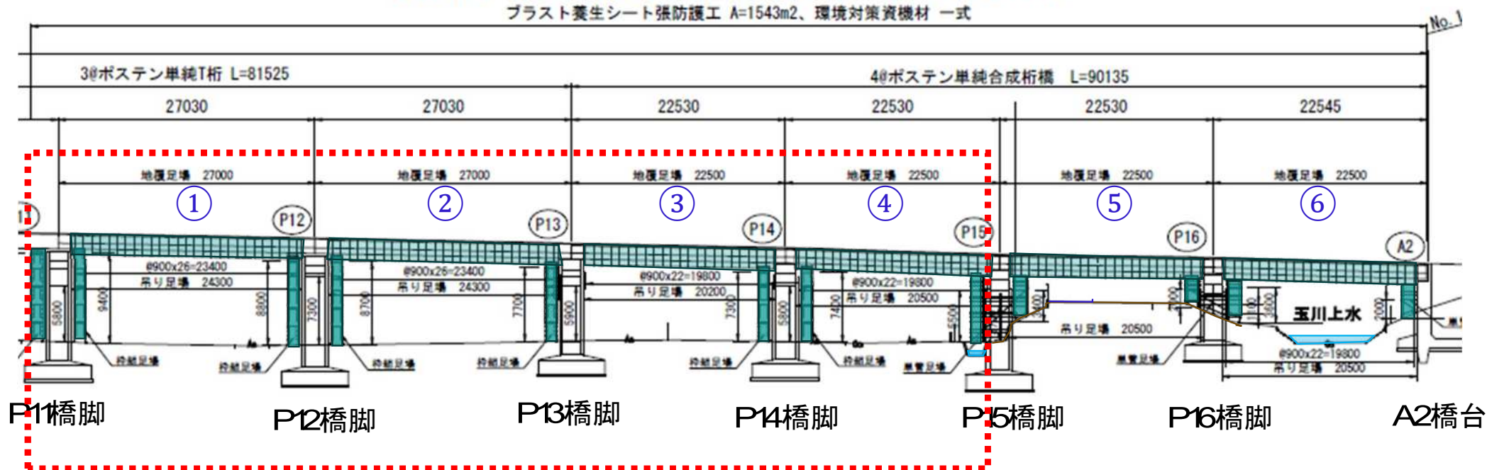
測面図
