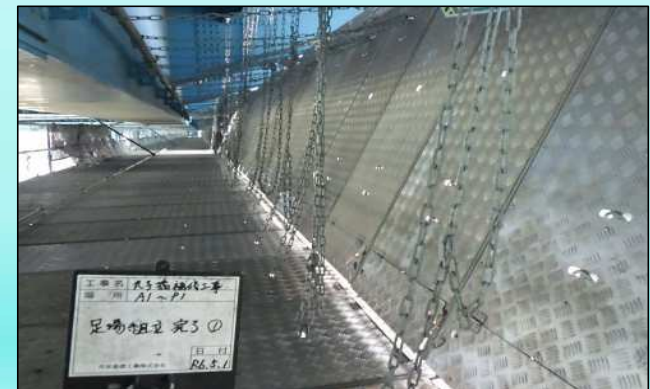
足場設置例（吊り足場）
