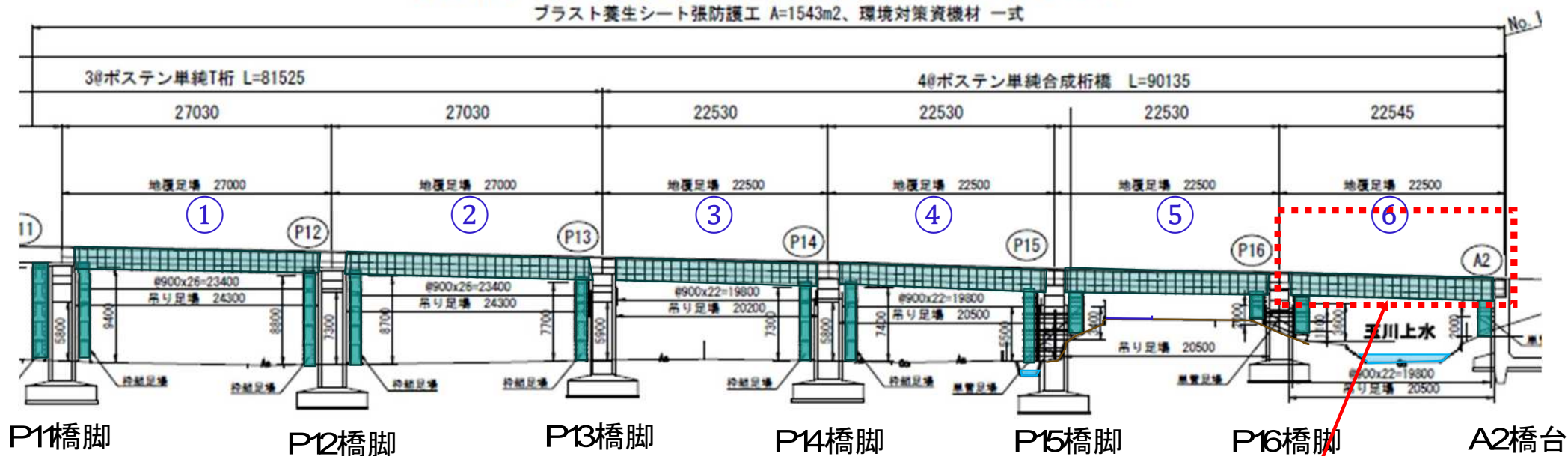
側面図
