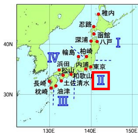
図 2-4 海面水位上昇の領域区分※2
