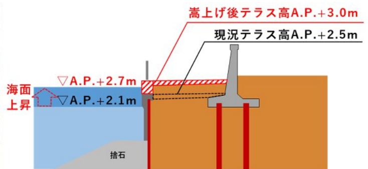
図 4-4 今後のテラス整備のイメージ
