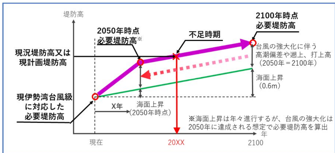
図 3-3 堤防高さが不足する時期の考え方
