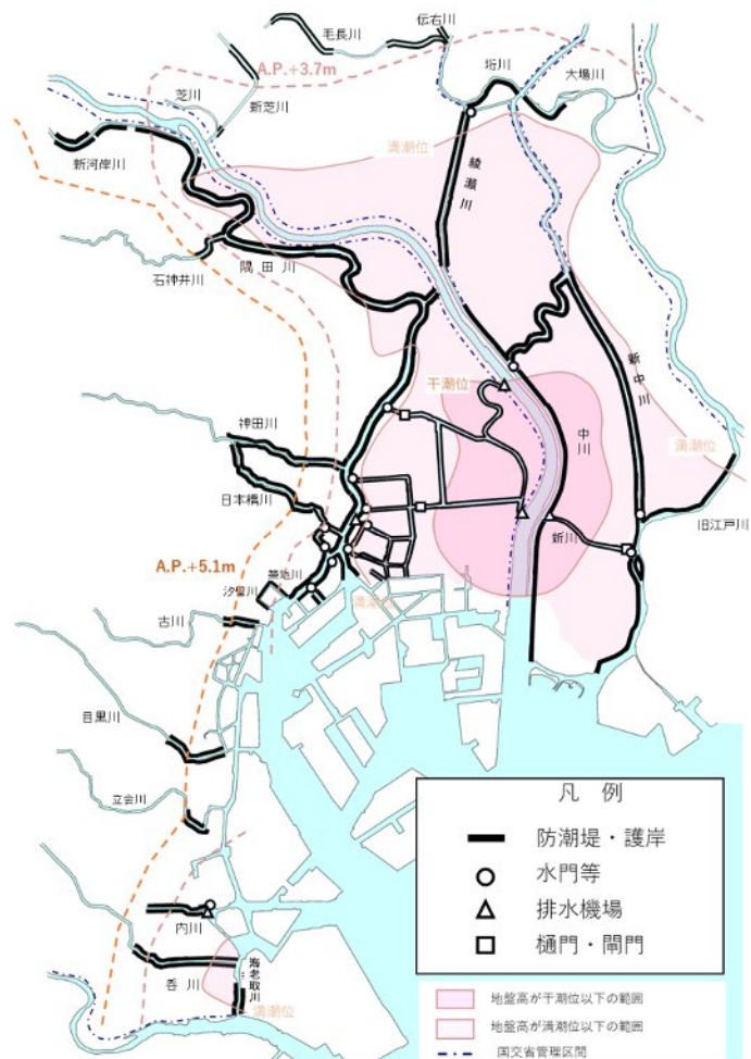
図 1-2 高潮防御施設整備箇所図
