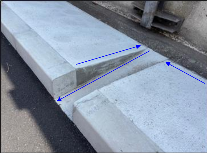
排水性を確保するため街渠にスリットを設けた。
