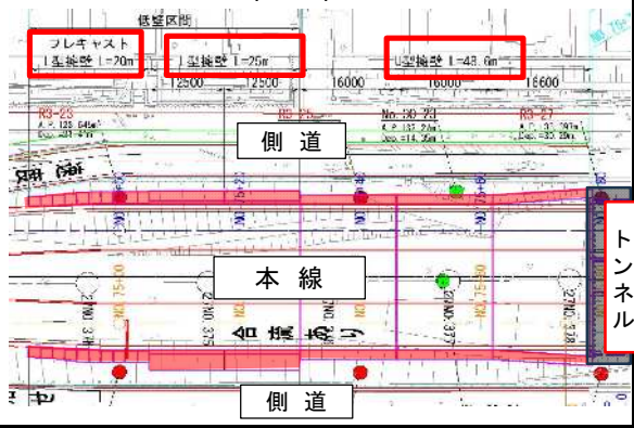
○委託対象構造物(一部)
