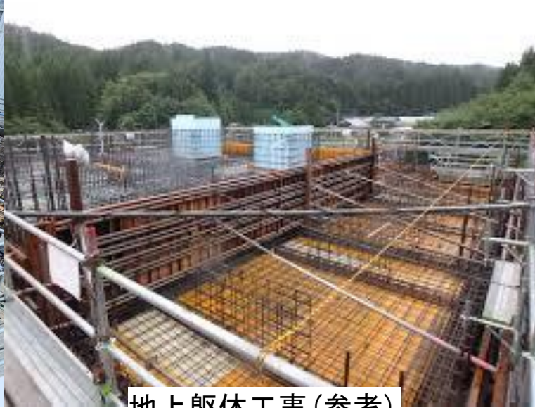
地上躯体工事(参考)
