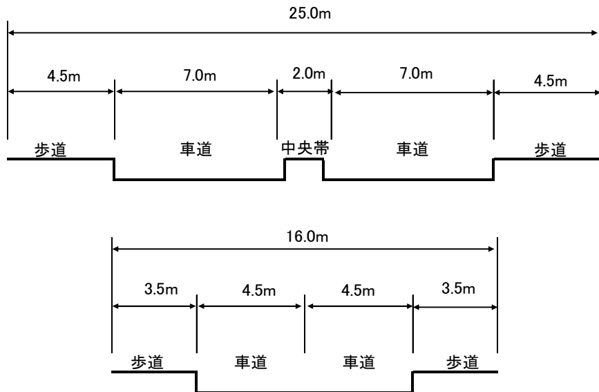
計画標準断面
