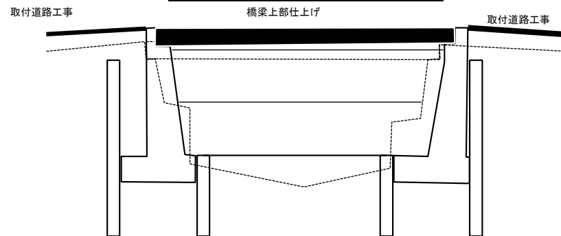
標準断面図 (新柳橋)
