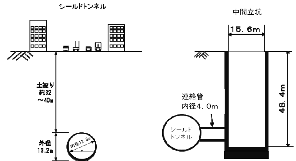
標準断面図
