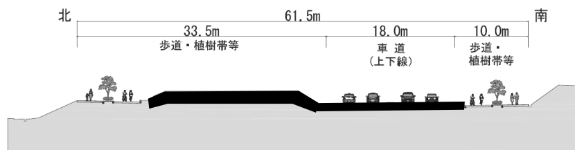
計画図
