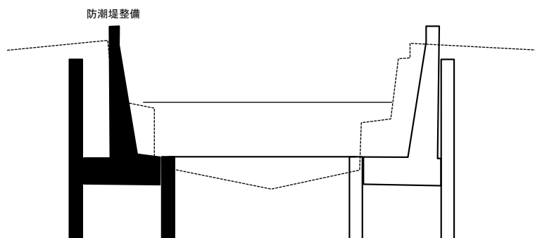
標準断面図 (新柳橋下流左岸)
