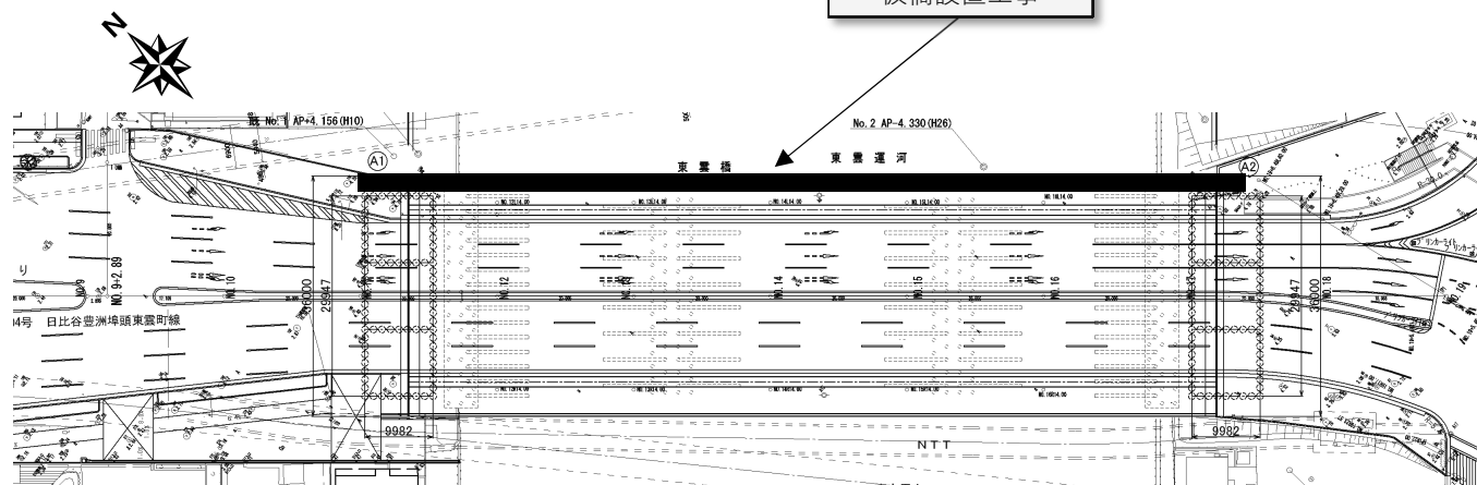
平面図
