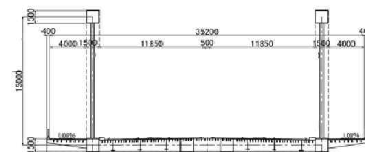
断面図
