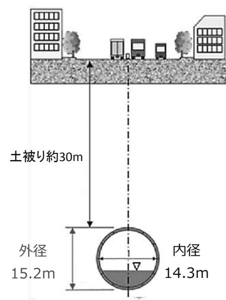
標準断面図
