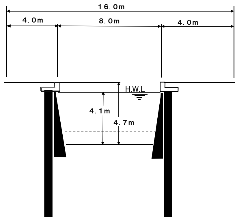
標準断面図
