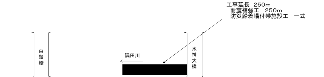
平面図
