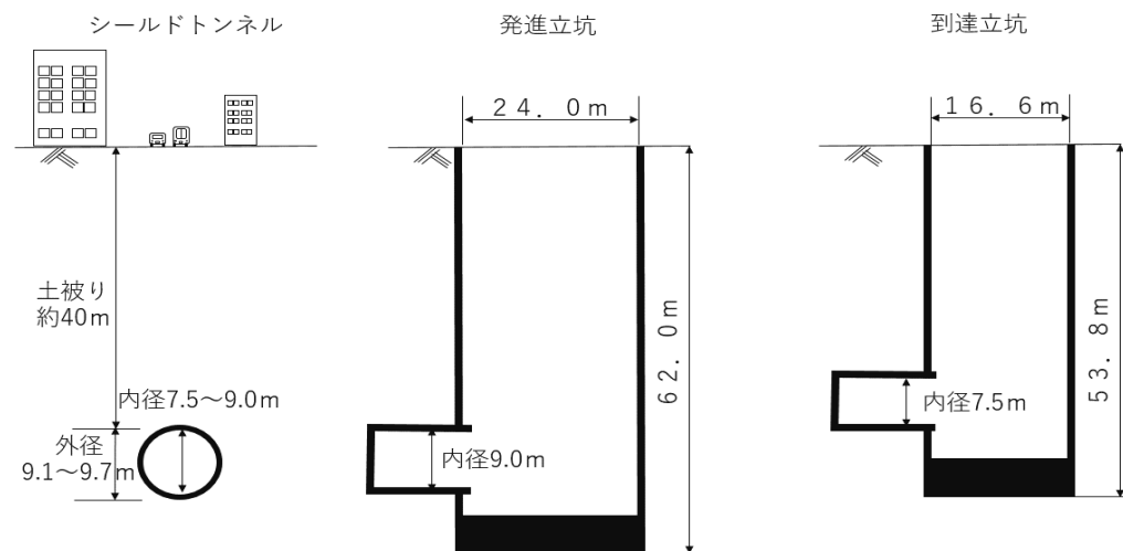
標準断面図
