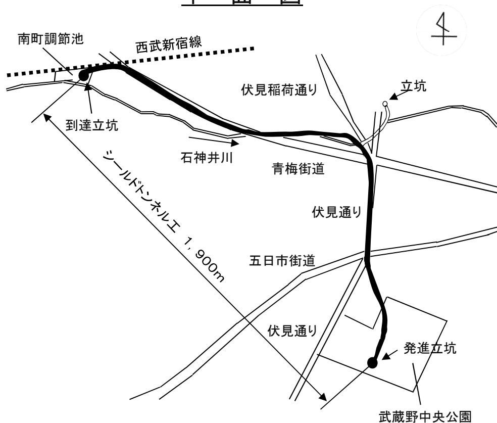
平面図
