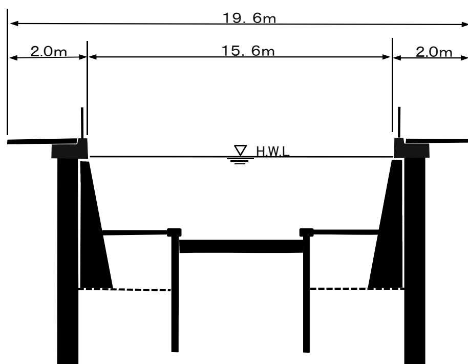
標準断面図
