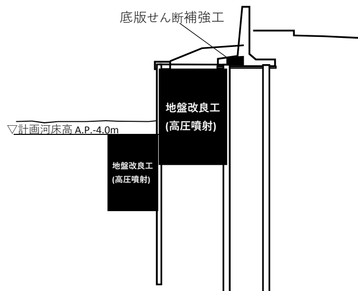
標準断面図
