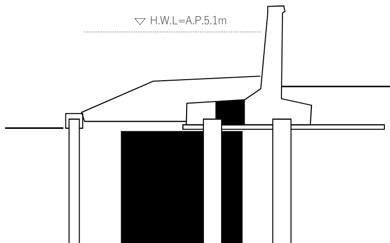
標準断面図
