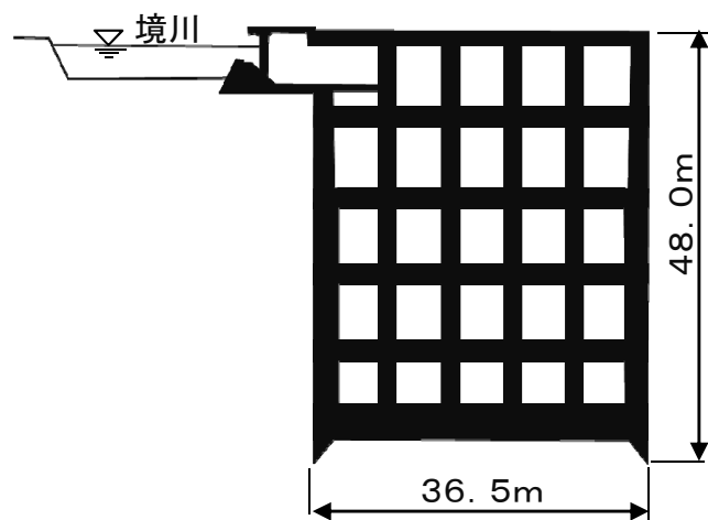
標準断面図
