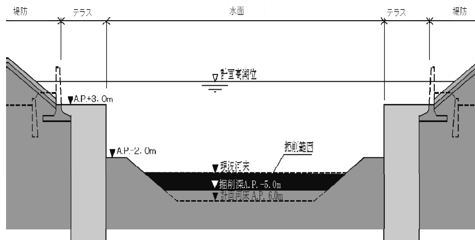
標準断面図
