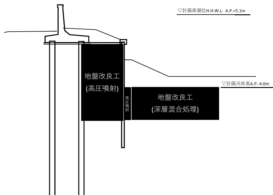
標準断面図
