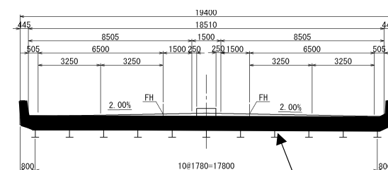
断面図
