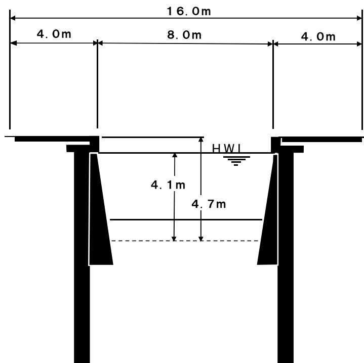
標準断面図
