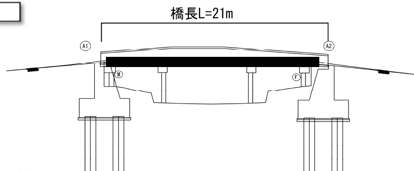
側面図
