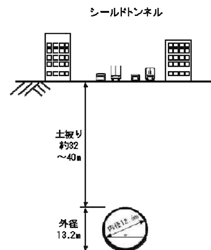
標準断面図
