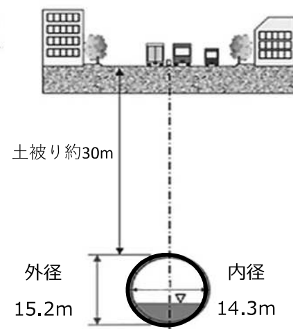
標準断面図
