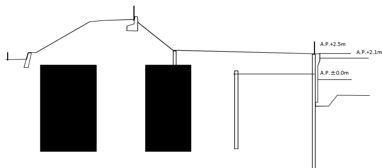
標準断面図
