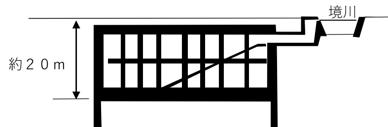
標準断面図
