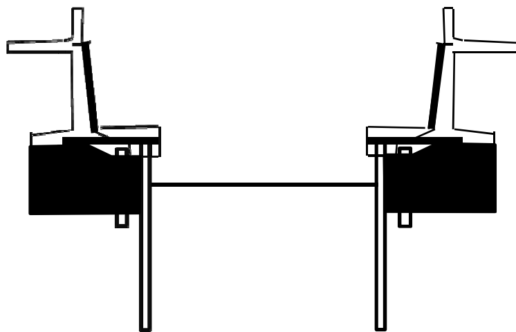
標準断面図
