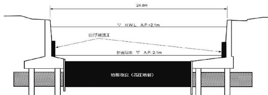
標準断面図
