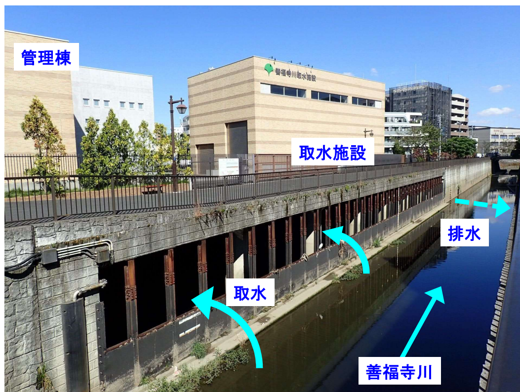
環状七号線地下調節池（善福寺川取水施設） 25
