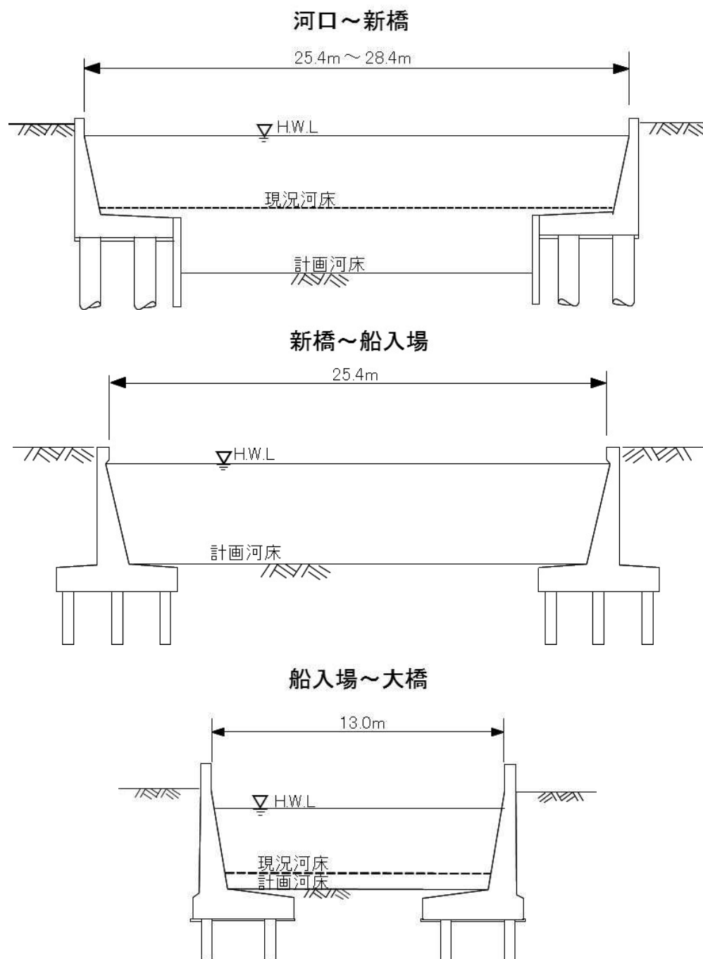
図 4-2 標準断面図
