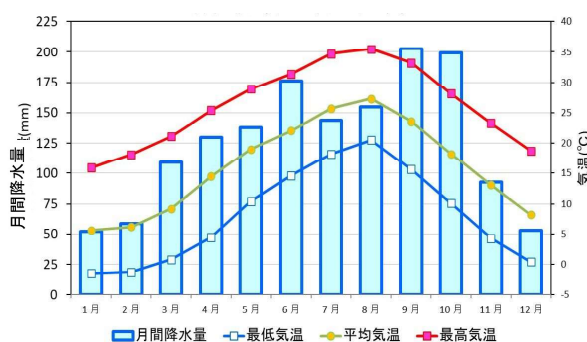
図 1-4 東京の年間降水量、気温の変化 (1961~2021 年)
