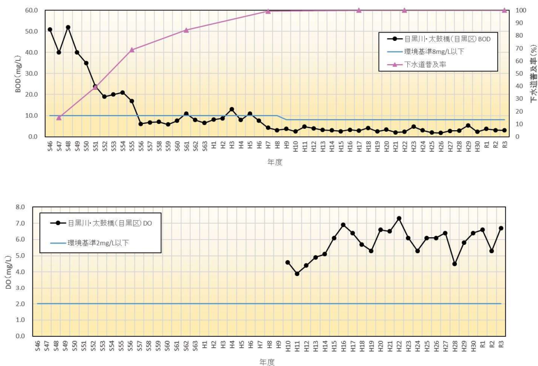
図 2-8 目黒川（太鼓橋）の水質の経年変化
