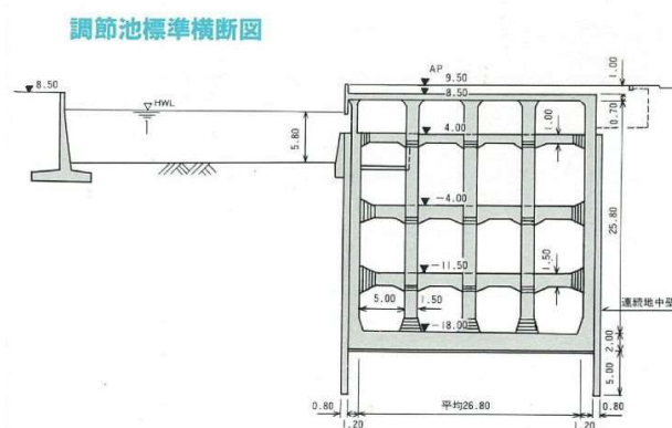
図 2-1 船入場調節池の標準横断面図
