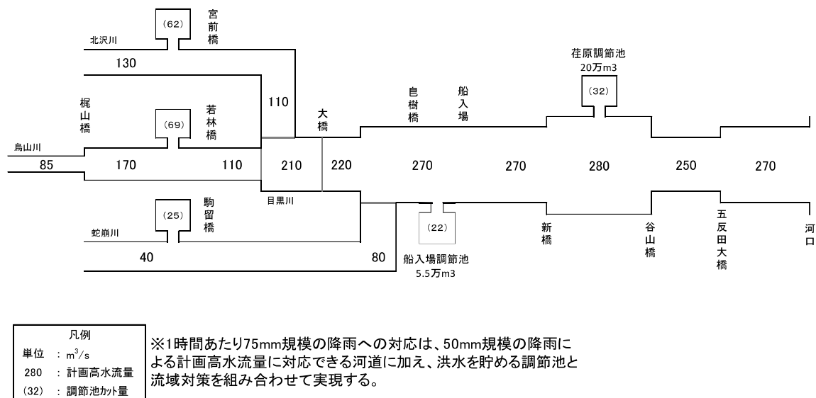
図 3-1 目黒川計画流量配分図
