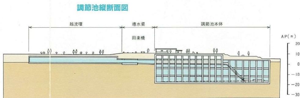
図 2-2 船入場調節池の縦断面図
