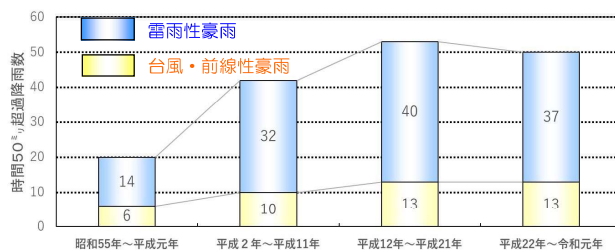
図 1-7 1時間50ミリを超える 発生要因別降雨数の経年変化 (昭和55年~令和元年(過去40年間))
