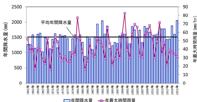
図 1-5 東京の年間降水量、最大時間雨量経年変化 (1961~2021 年)
