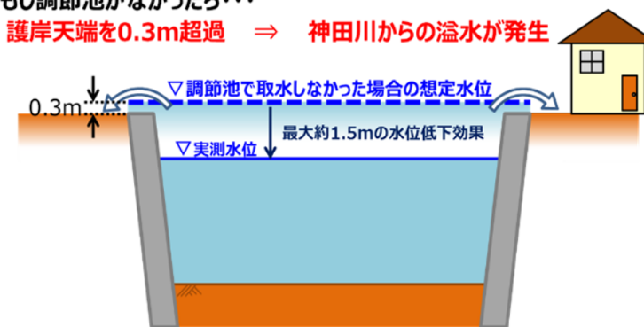
神田川の水位断面イメージ
