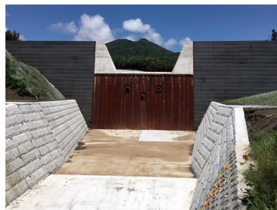
砂防堰堤(大島町差木地沢)
