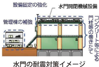
水門の耐震対策の様子(上平井水門)
