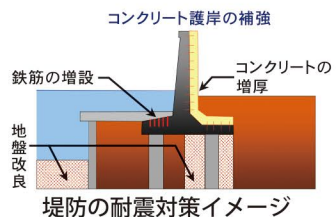
堤防の耐震対策の様子(隅田川)
