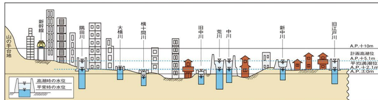
東部低地帯の地盤高
