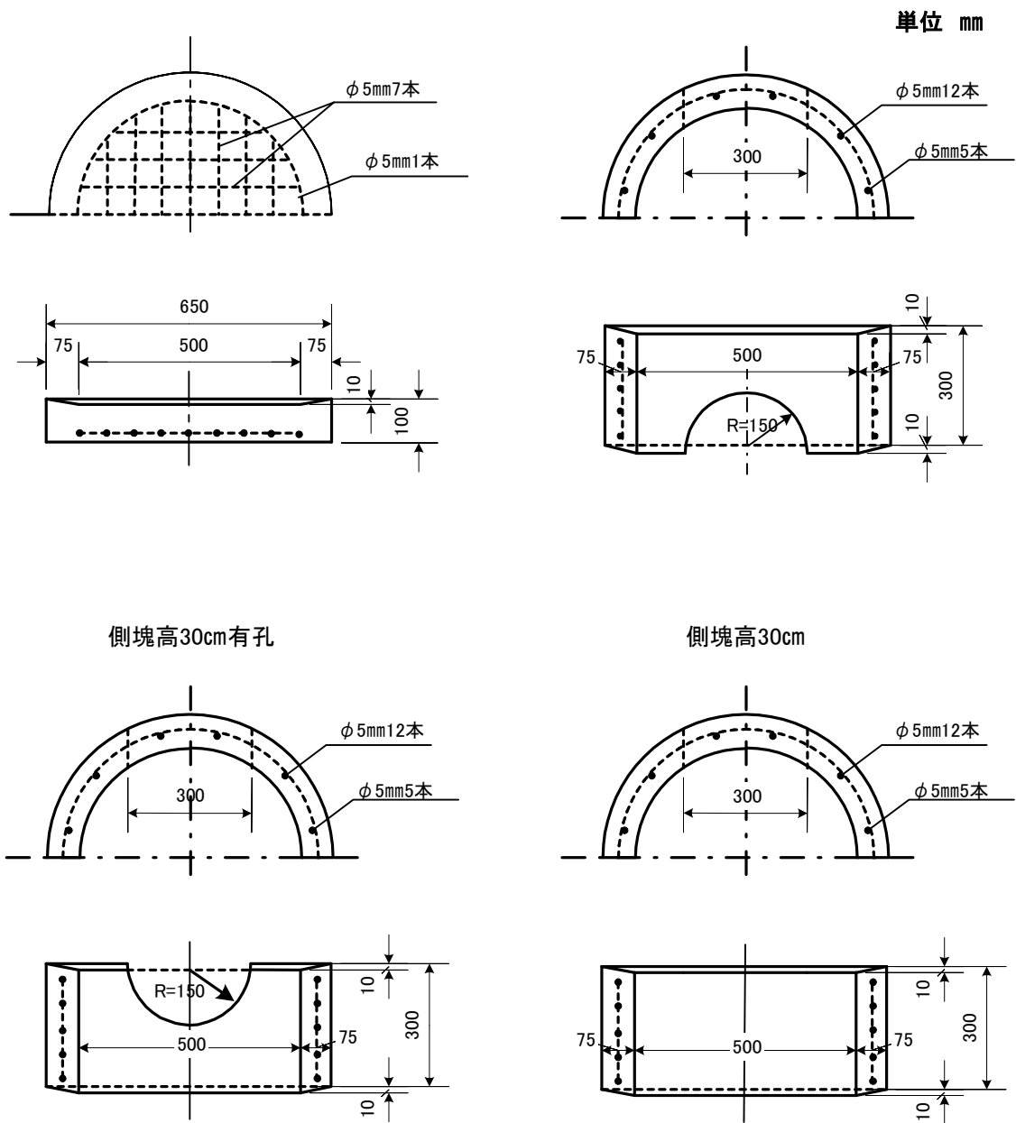
図 327-4 街きょ用集水ます側塊・底版塊
