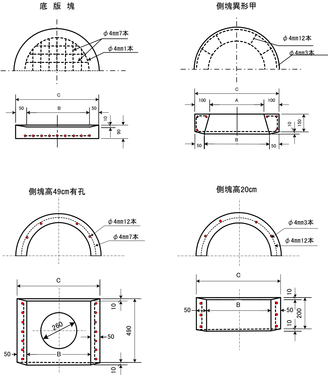
図 327-6 L形用集水ます側塊・底版塊
