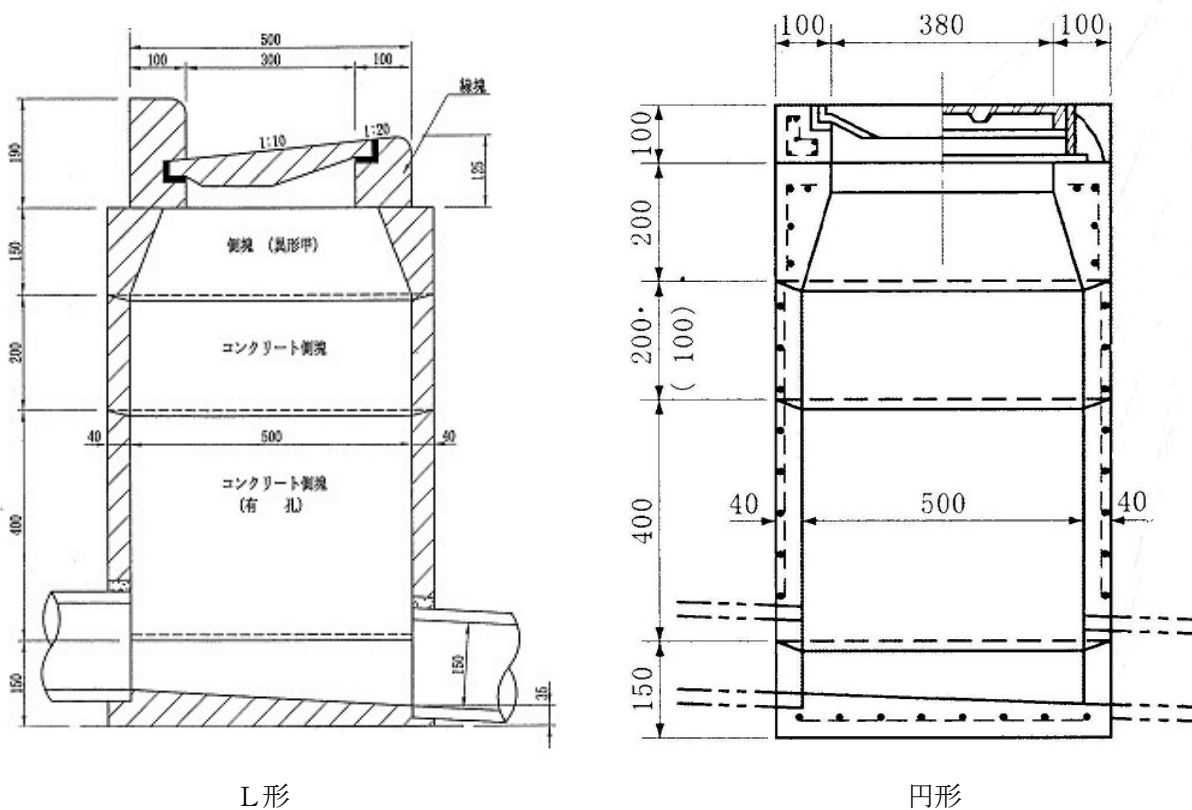
図 329-1 組 立 図
