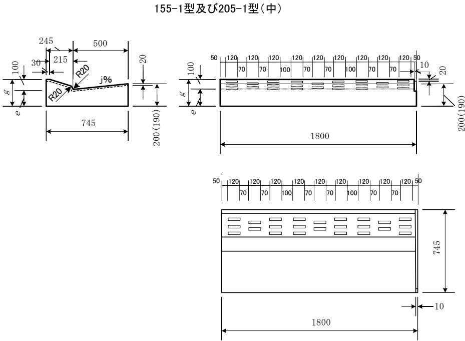
155-1型及び205-1型(基礎コンクリート版)
