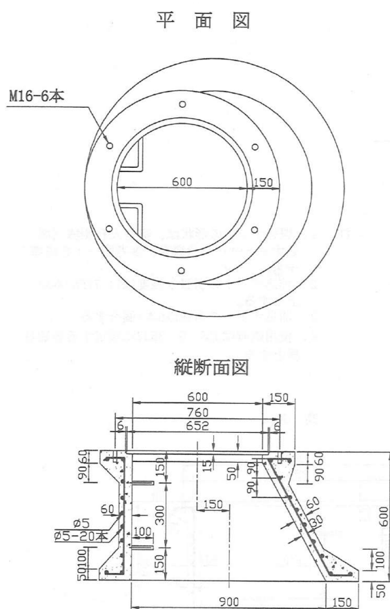
图 330-2 円形片斜壁人孔側塊
