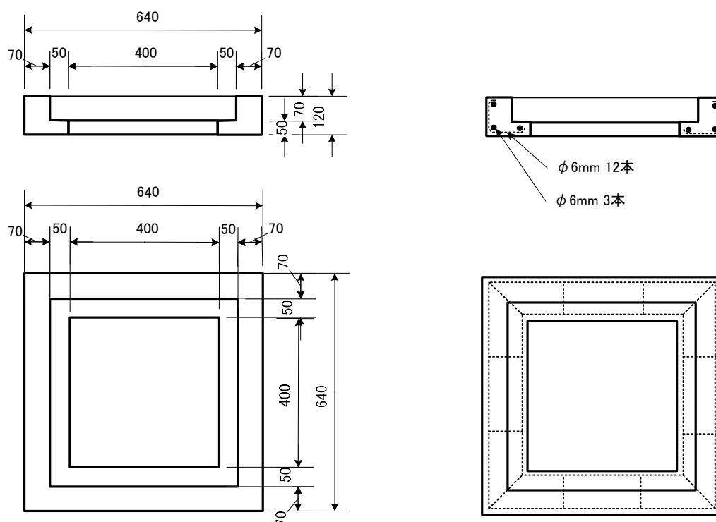
図 327-7 U形用集水ます縁塊
