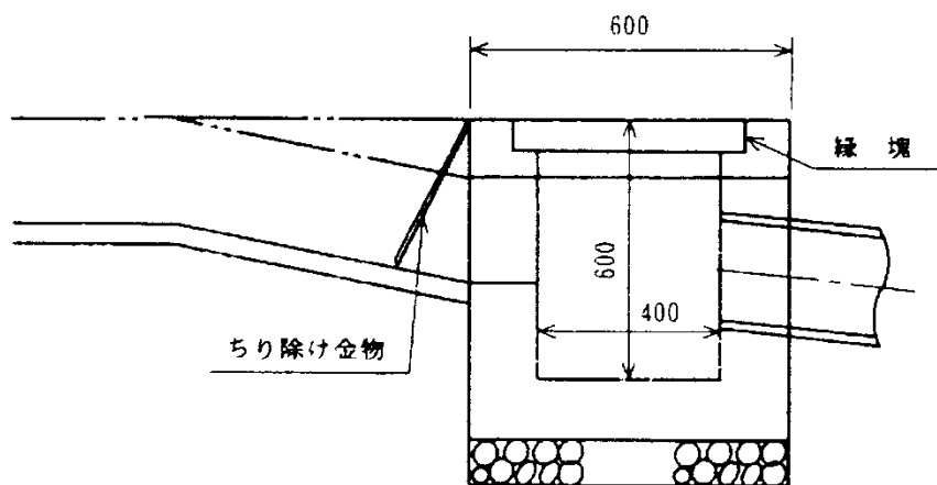
U形用集水ます
