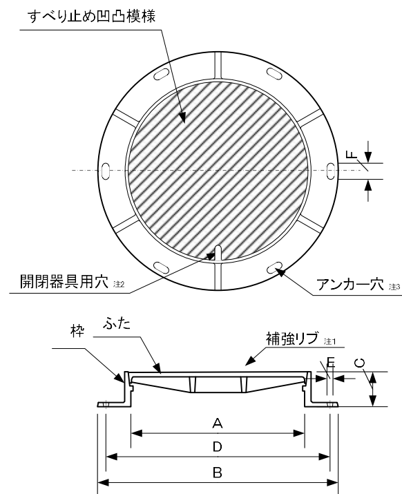
図 332-1 鑄鉄製ふた
