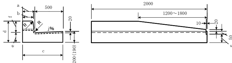
図 345-4 (歩行者横断用)
