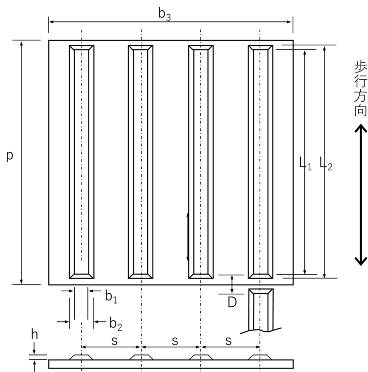
図 316-3 線状ブロックの形状・寸法及び突起の配列
