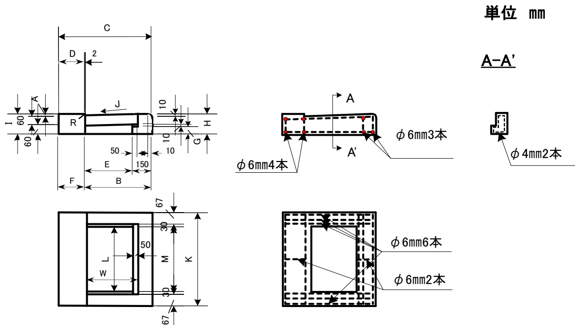
図 327-3 街きょ用集水ます縁塊（歩行者横断用切下げ部）
