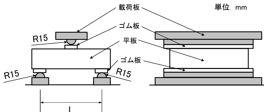
図315-1 曲げ耐力試験方法
