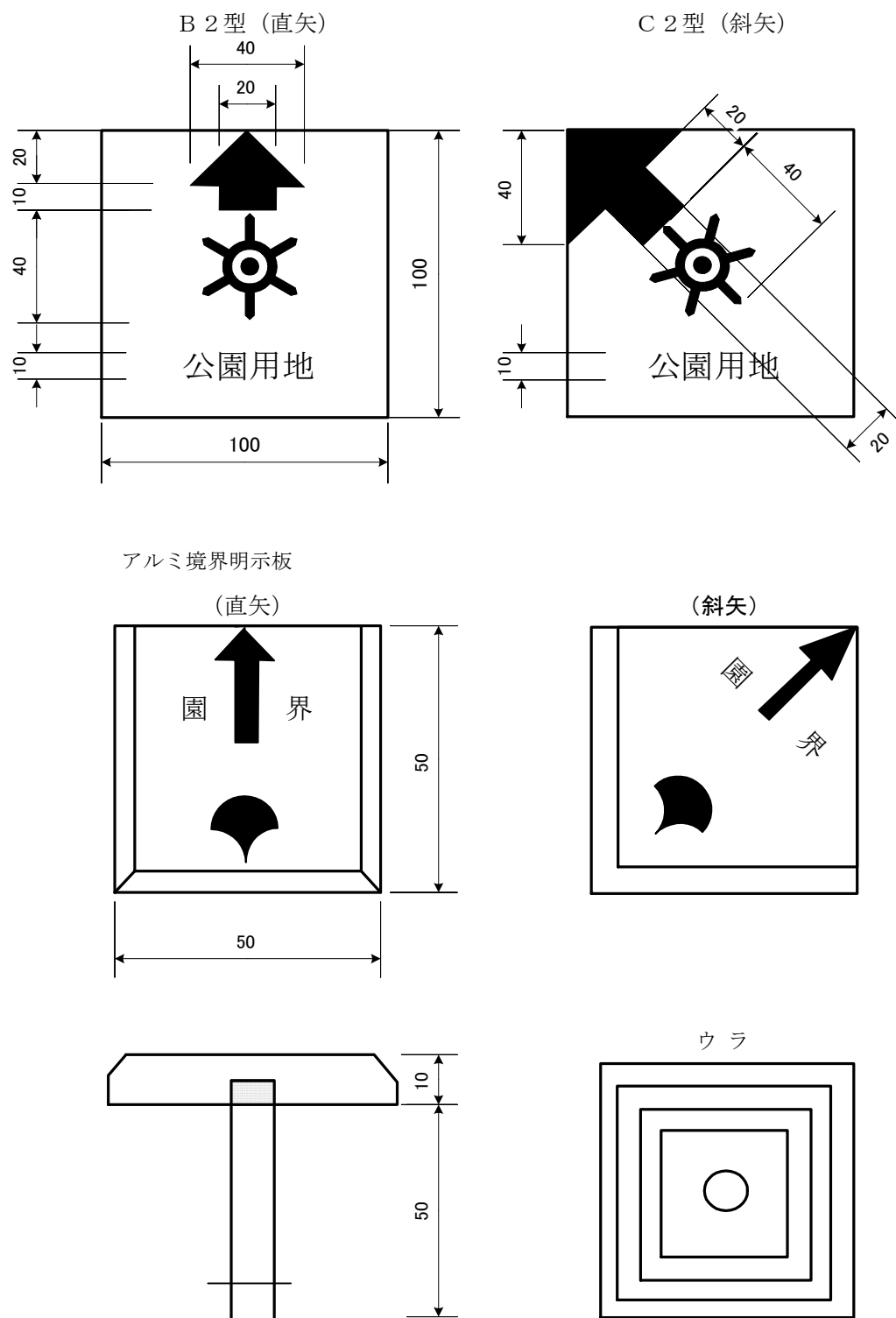
図337-2 公園用境界標杭
