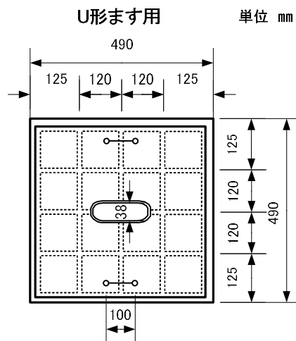
図 327-9 装鉄製ふた
