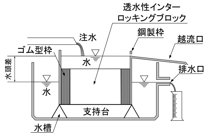
図317-6 透水試験
