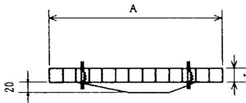
図 328-1 格子ふた
