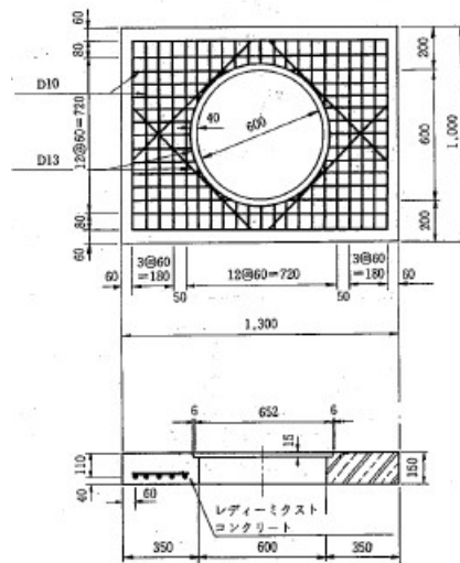
図 331-1 矩形床版塊
