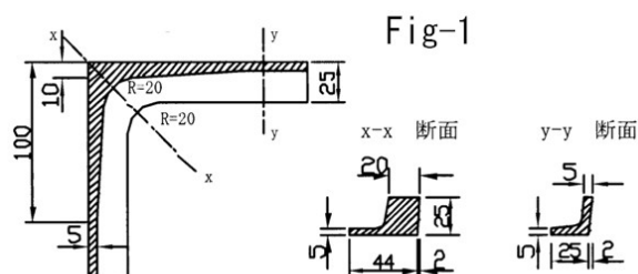
図 329-4 L 形汚水ます用ふた
