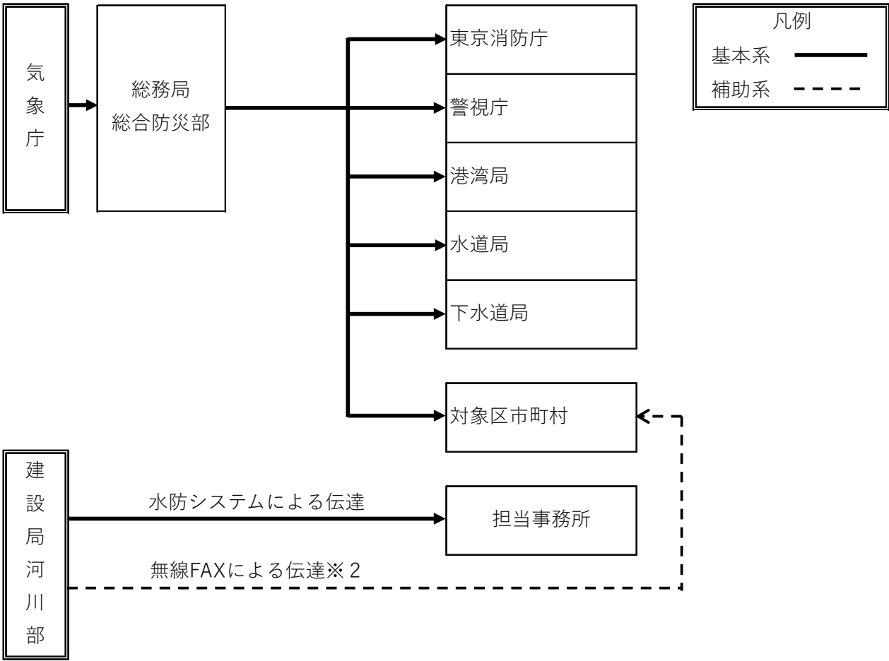
(5) 伝達系統図
