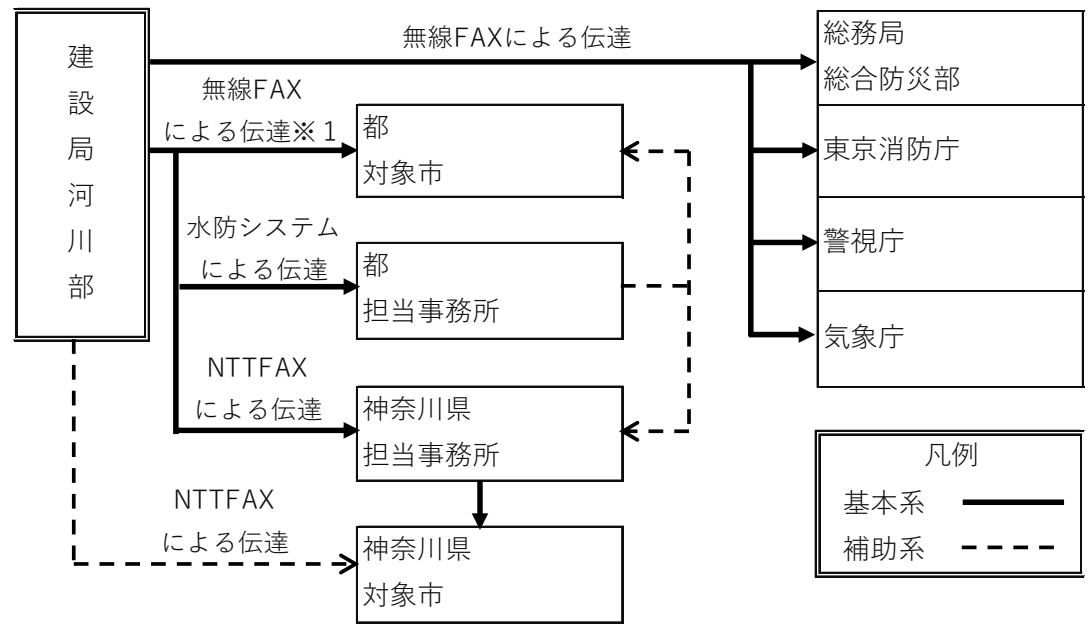
(5) 伝達系統図
