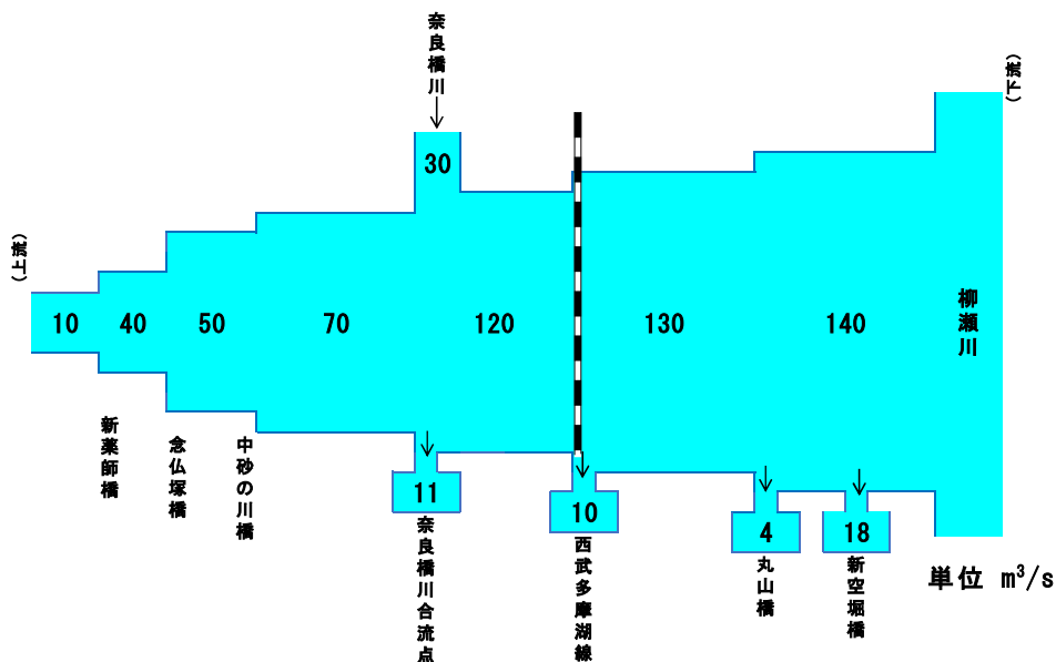
図 3-2 空堀川の流量配分図
