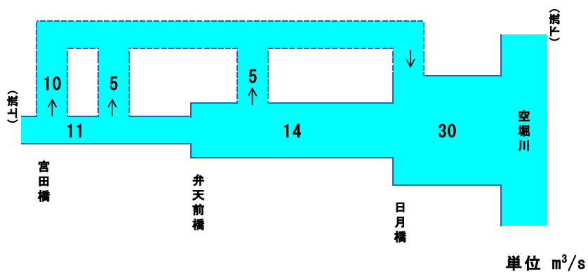
図 3-3 奈良橋川の流量配分図
