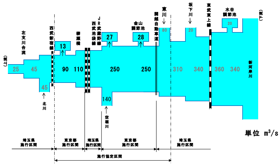
図 3-1 柳瀬川の流量配分図
