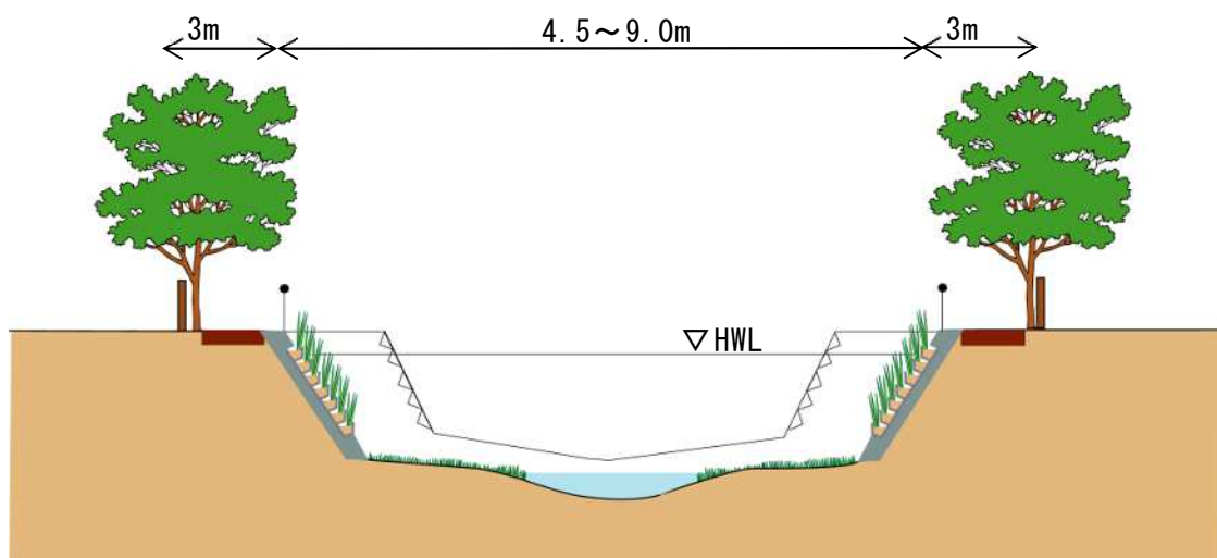
図 4-7 奈良橋川の標準横断面図
