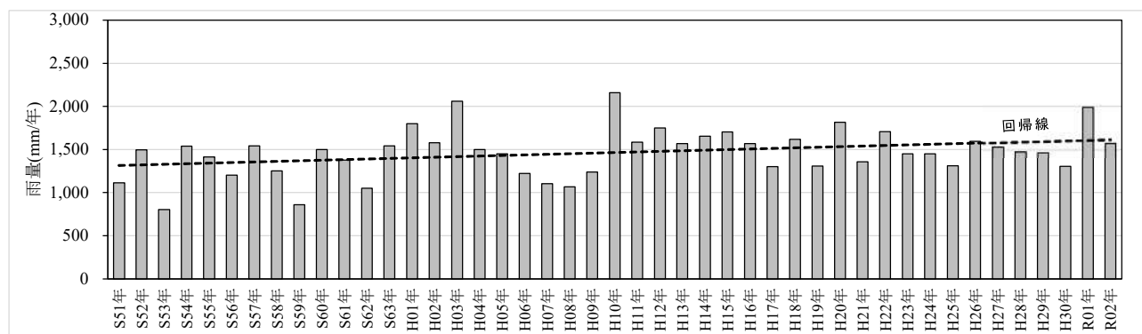
図 1-5 年降水量の経年変化(気象庁 所沢地域気象観測所)
