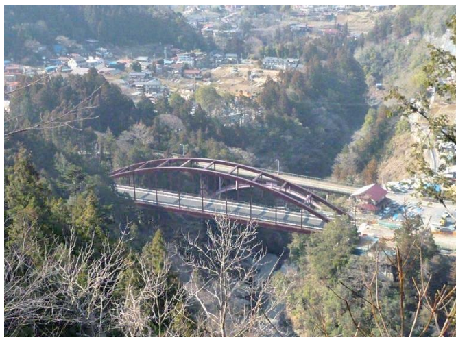
国立公園内のためこげ茶に着色した将門大橋（下路式鋼ローゼ橋）
