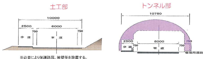
標準断面図(城山工区)
