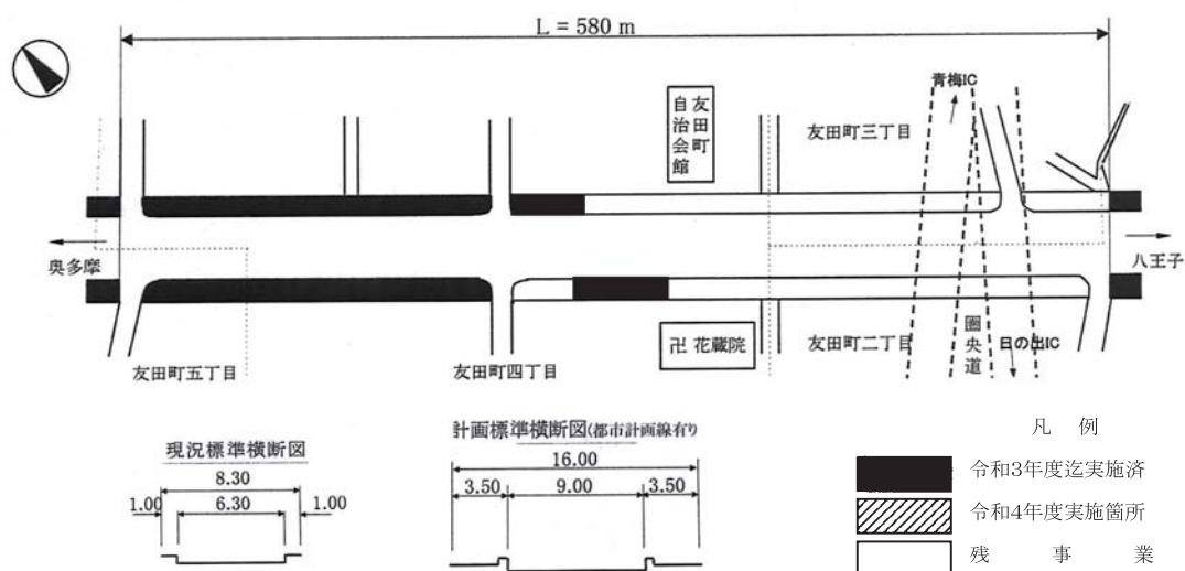
国道411号(友田二～五丁目地区)整備状況図
