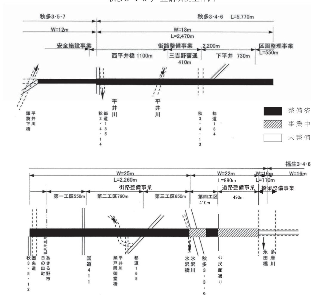
秋多3・4・6号 整備状況全体図
