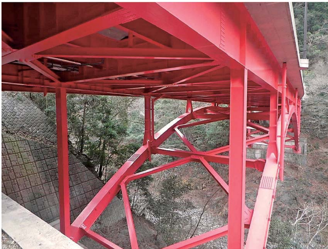
橋梁維持事業（愛宕大橋塗装） 「一般都道奥多摩あきる野線（第184号）多摩川南岸道路」 西多摩郡奥多摩町氷川地内 平成31年2月完成
