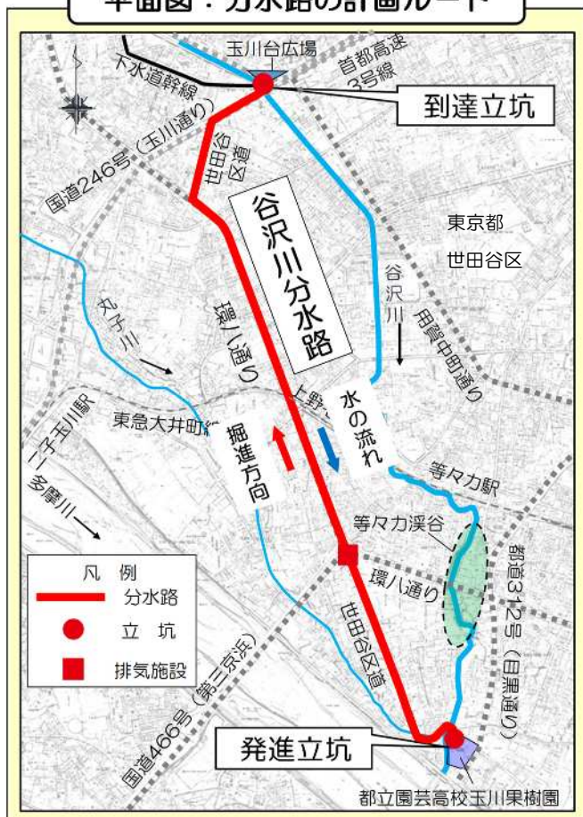
平面図：分水路の計画ルート
