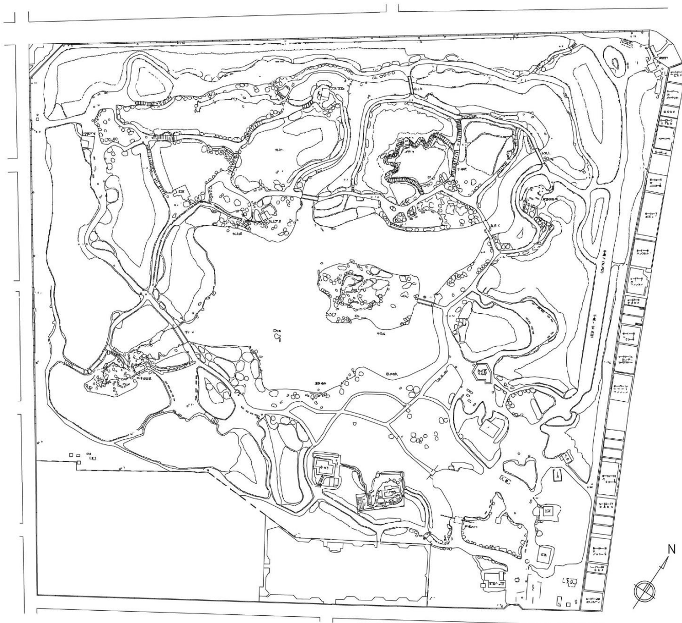
図2-39 「六義園施設測量 施設平面図」平成11（1999）年 東京都建設局
