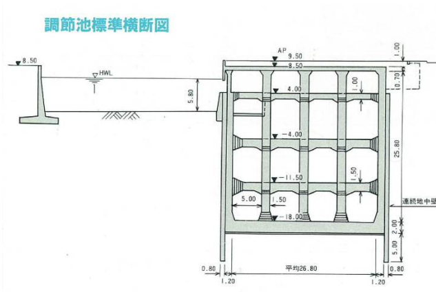
図 2-1 船入場調節池の標準横断面図
