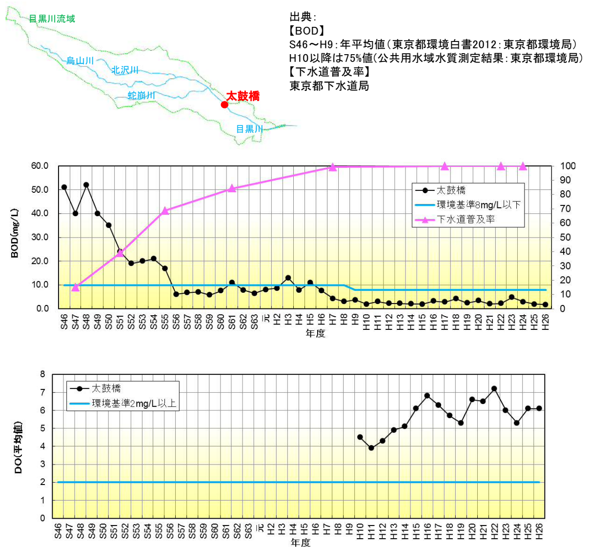
図 2-8 目黒川（太鼓橋）の水質の経年変化
