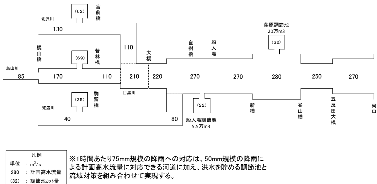
図3-1 目黒川計画流量配分図
