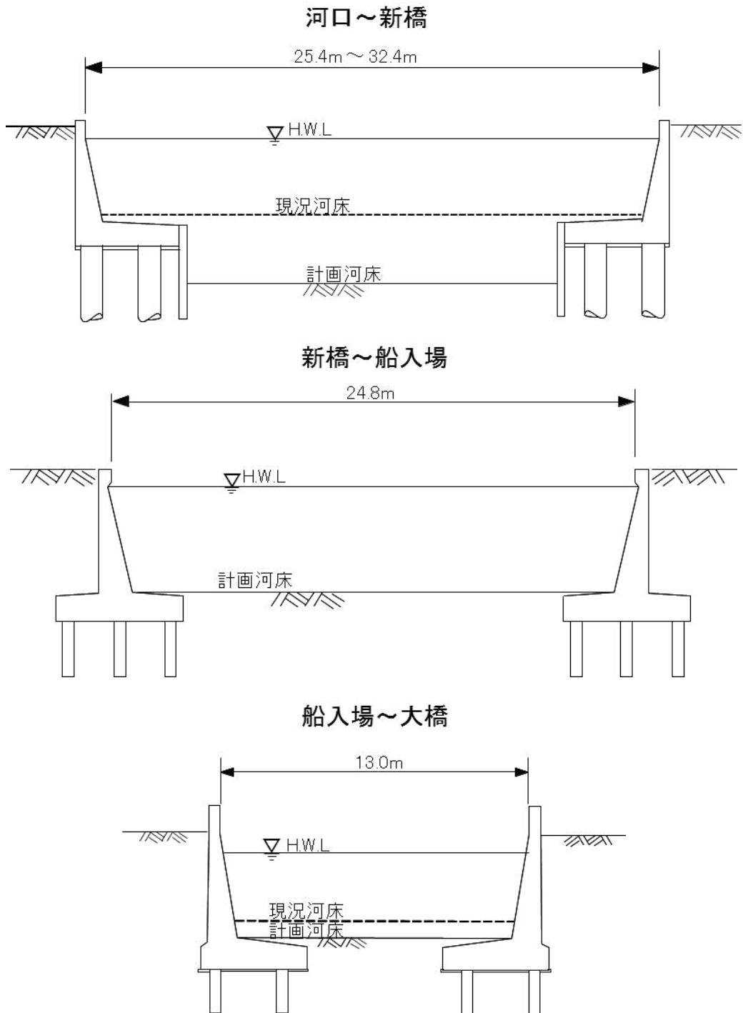
図 4-2 標準断面図
