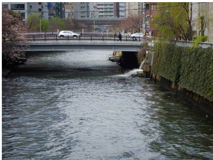
写真 2-4 地下鉄からの湧水放流状況
