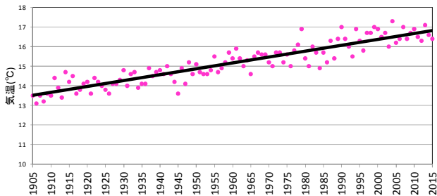
図 1-6 東京の年平均気温経年変化 (1905~2015年)
