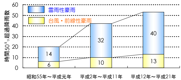
図 1-7 1時間50ミリを超える発生要因別降雨数の経年変化 (昭和55年~平成21年(過去30年間))
