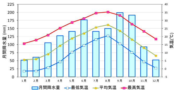
図 1-4 東京の年間降水量、気温の変化 (1961~2015年)
