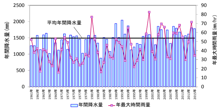
図 1-5 東京の年間降水量、最大時間雨量経年変化 (1961~2015年)
