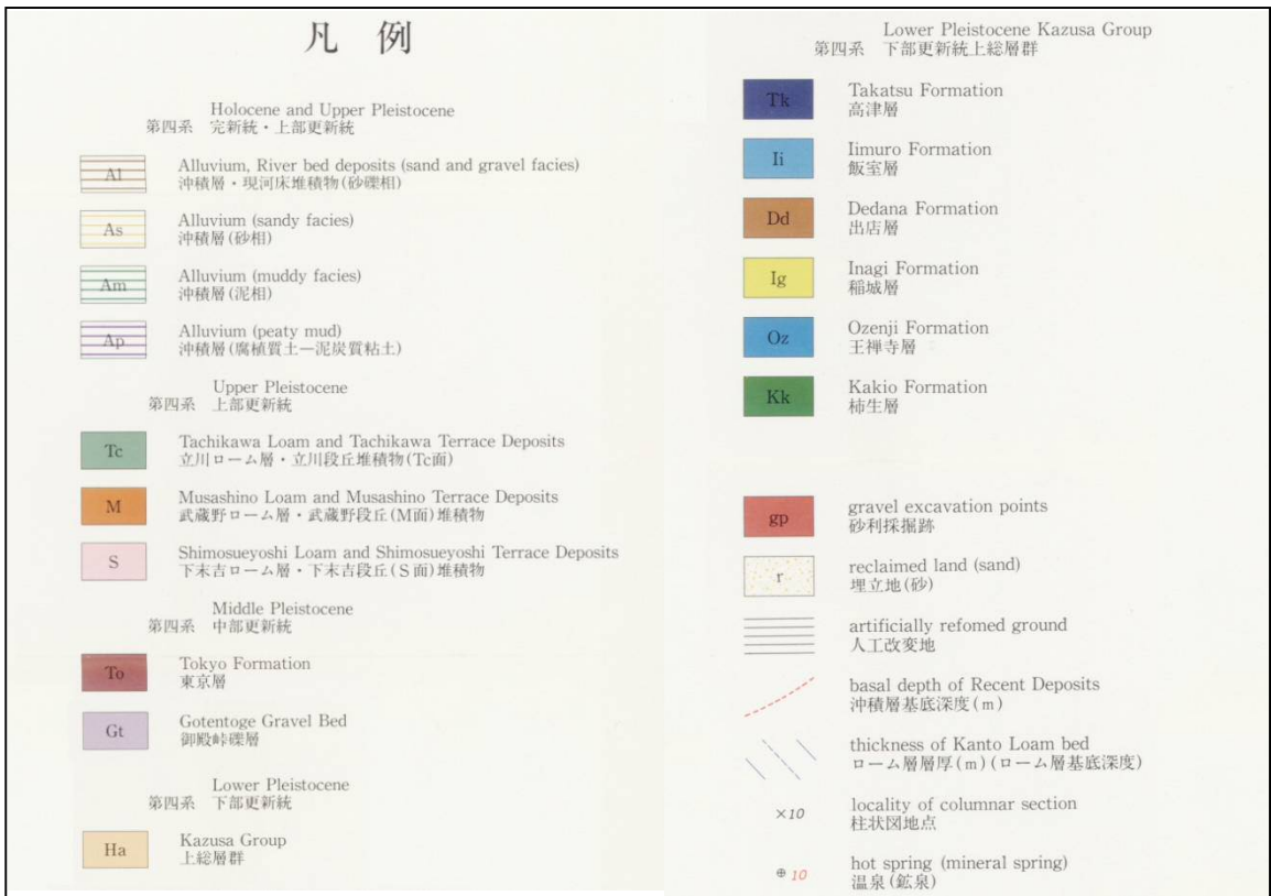
図 1-2 目黒川周辺の地質平面図
