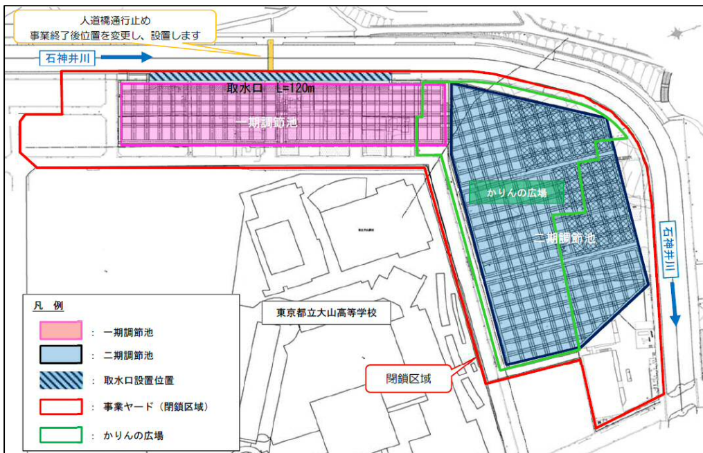
城北中央公園調節池 施工図
