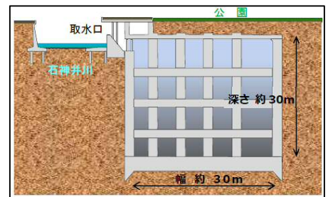
調節池断面イメージ
