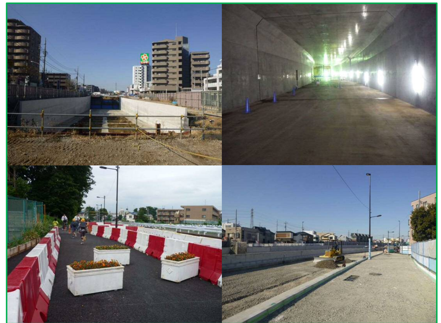
(左上) 平和台掘割部 (右上) ボックスカルバート完成部 (左下) 暫定歩道開放状況 (右下) 街築工事施工状況
