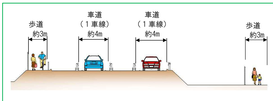
交通開放イメージ図（B-B）
