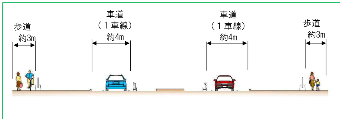
交通開放イメージ図（A-A）
