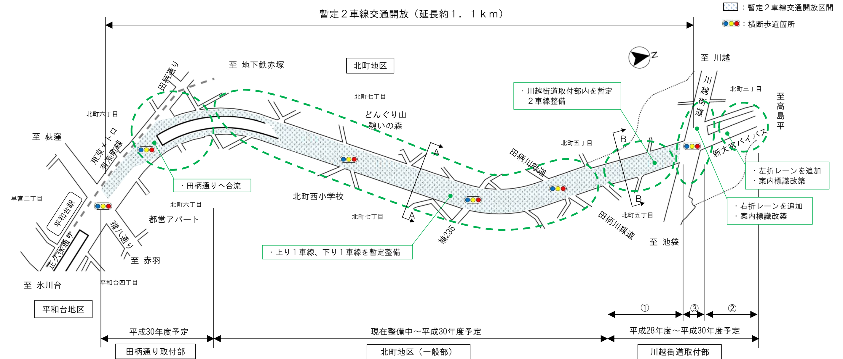
交通開放イメージ図（A-A）
