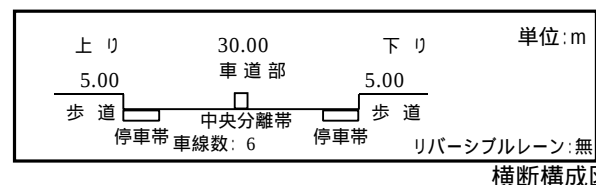
横断構成図
