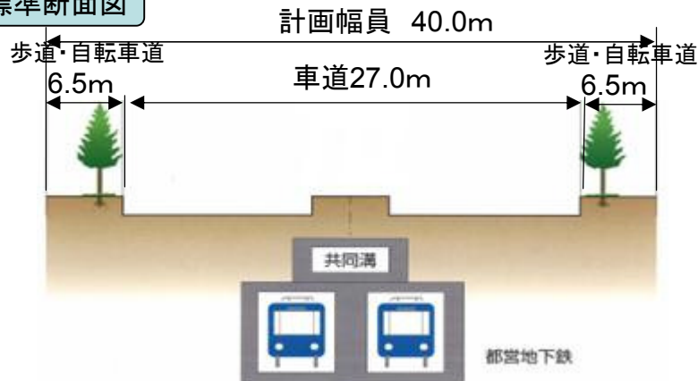
標準断面図
