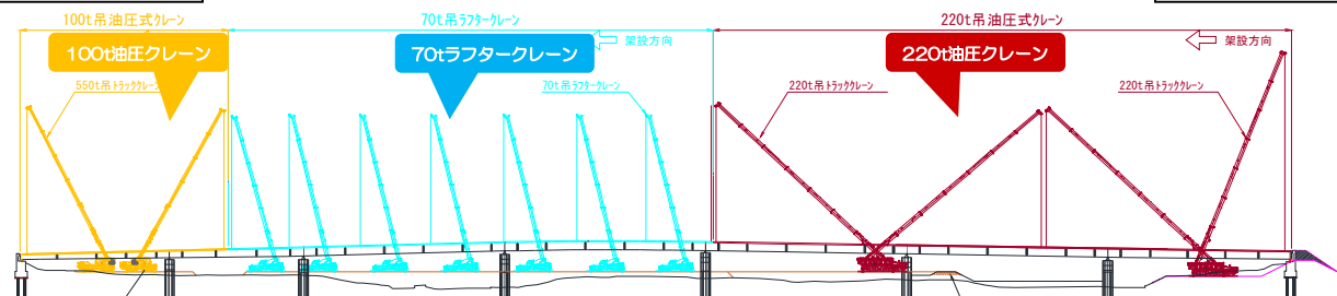
パネル敷設側面図
