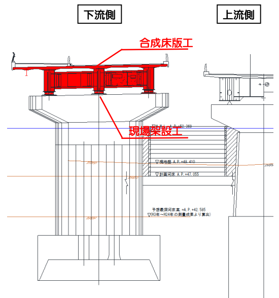
断面図
