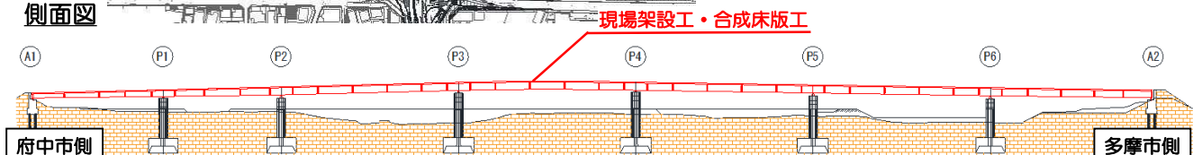
側面図
